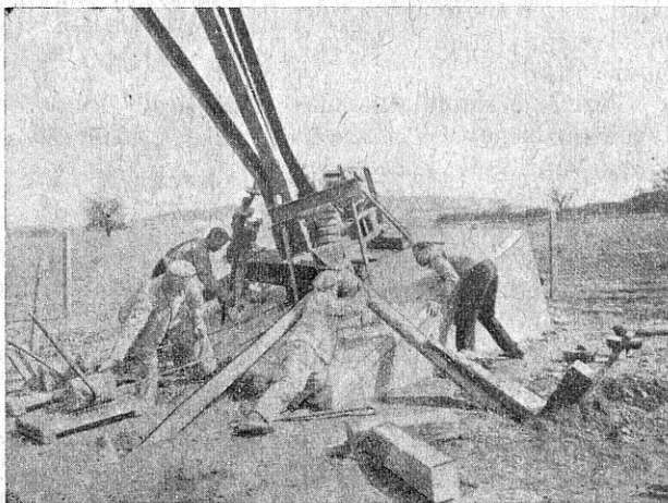
ANTENNIMASTI „JALAHÄIGUSE“ ARSTIMINE Sottensi raadiojaam pidi hiljuti oma antennimasti jalga parandama. Ta tösteti hüdrauliste vintide abil üles, et pääseda vigastatud koha juure.
