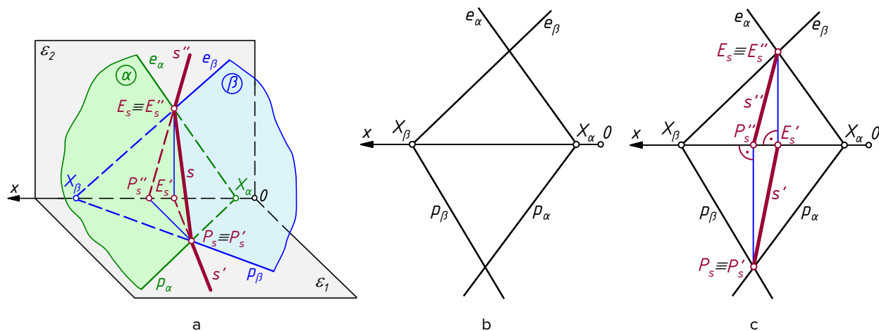
Joonis 3.56. Jälgedega antud tasandite lõikesirge tuletamine: a – piltkujutis; b – lähteandmed; c – lahendus kaksvaatel.
