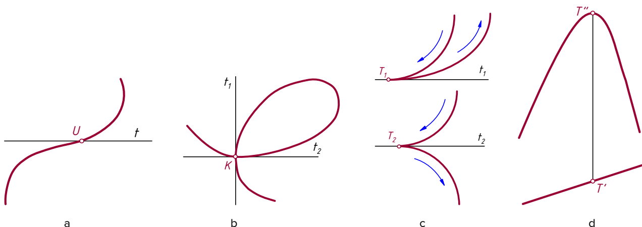
Joonis 3.125. Kõverjoonte iseäraseid punkte: a – käänupunkt; b – sõlmpunkt; c – tagasipõördepunkt; d – haripunkt.
