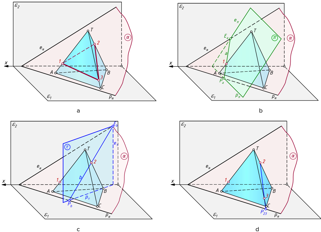
Joonis 3.117. Püramiidi ja üldasendilise tasandi lõikumise ülesande etapiviisiline lahendamine (piltkujutis).
