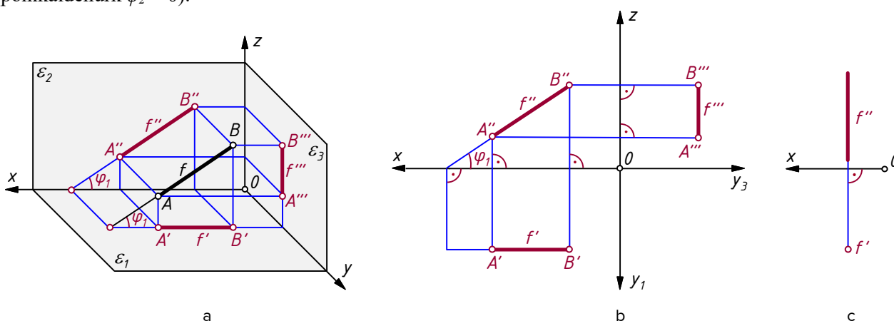
Joonis 3.21. Frontaal: a - frontaali piltkujutis; b - frontaali kolmvaade; c - frontaali erijuht f \perp \varepsilon_1 .
