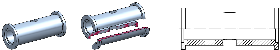
Joonis 4.56. Poolvaatlõige.
