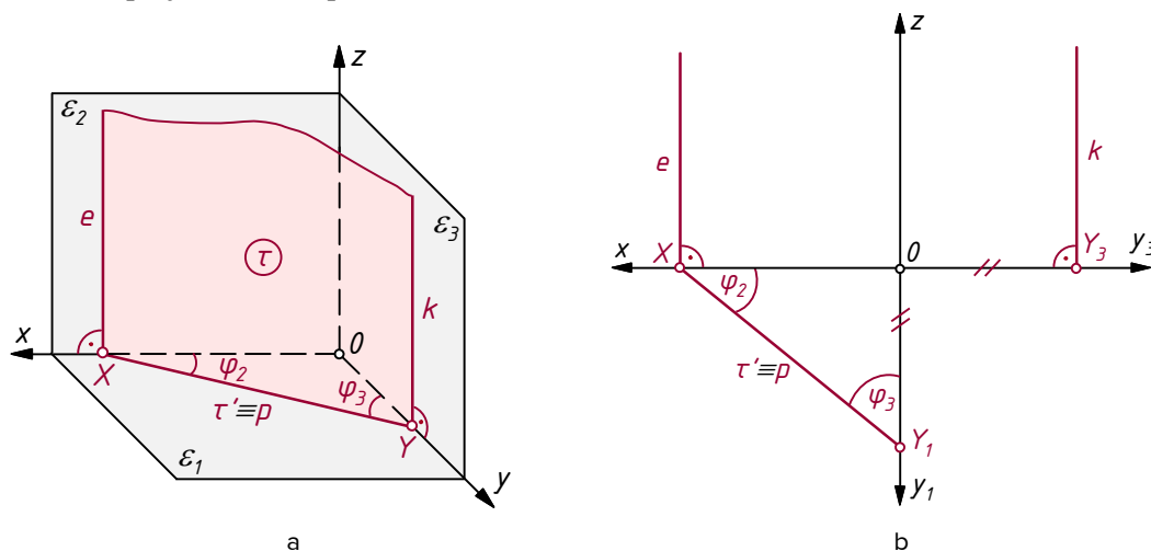
Joonis 3.40. Põhiekraani risttasand: a – piltkujutis; b – kolmvaade.
