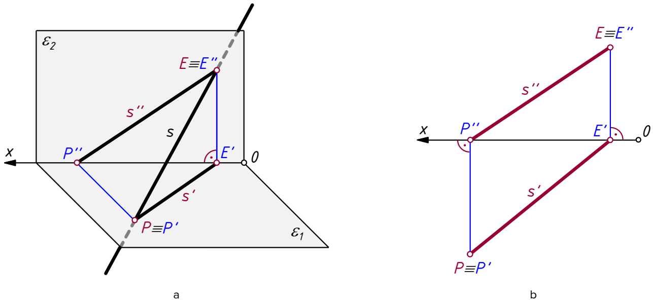
Joonis 3.34. Sirgjoone jälgpunktid: a – piltkujutis; b – sirgjoone jälgpunktide P ja E tuletamine kaksvaatel.
