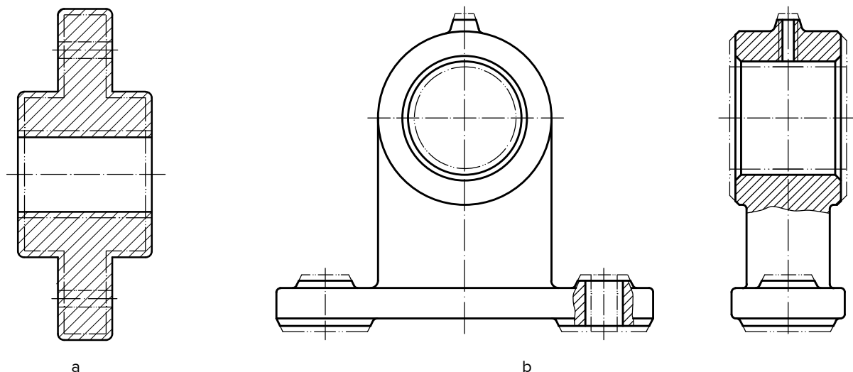
Joonis 4.41. Detaili kuju toorikul (a) ja tooriku kuju detaili tööjoonisel (b).
