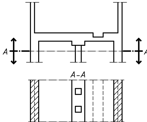
Joonis 4.12.b. Peegeldatud ristprojektsiooni meetod.
