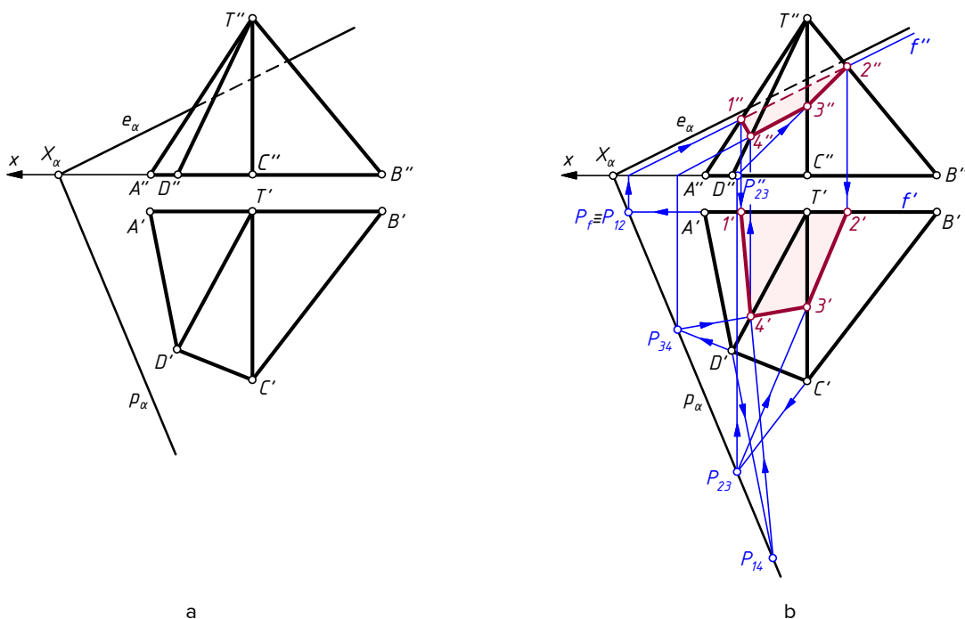
Joonis 3.120. Lõike kaksvaade tuletamine lisaekraani kasutamata: a – lähteandmed; b – lahendus kaksvaatel.
