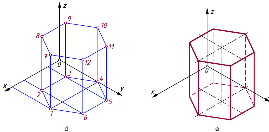
Joonis 3.105. (järg).
