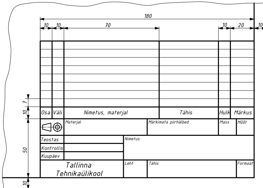
Joonis 4.180. Koostejoonisega ühildatud tükitabel.
