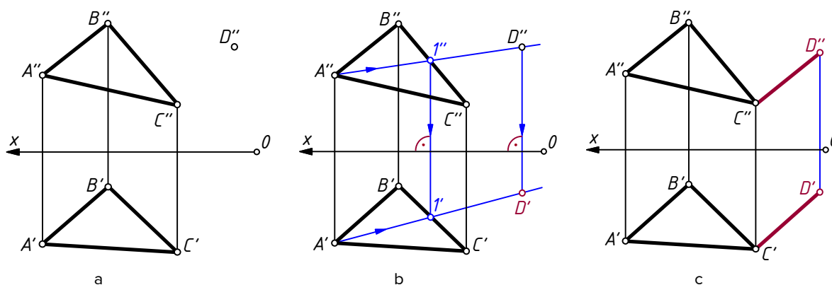
Joonis 3.47. Tasandil asetseva punkti (a, b) ja sirge (c) puuduva projektsiooni tuletamine: a – lähteandmed; b, c – lahendus kaksvaatel.
