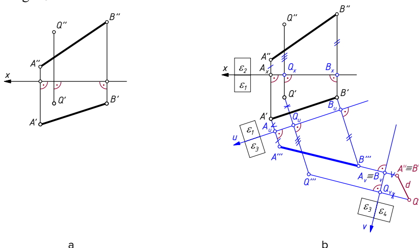
Joonis 3.83. Punkti kauguse tuletamine üldasendilisest sirgest lisaekraani abil: a – lähteandmed; b – lahendus.
