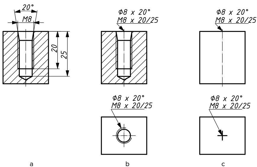
Joonis 4.132.6. Koonilise süvisega nurgaga 20° (puuritud ava läbimõõduni) 25 mm sügavusega ava keermega M8, kerme pikkus 20 mm. Ava põhi ei ole täpsustatud.
