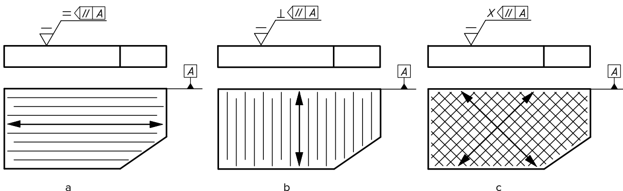
Joonis 4.144. Viitega kasutatavad pinnakihi konaruste sihi kujutised ja tähistus.
