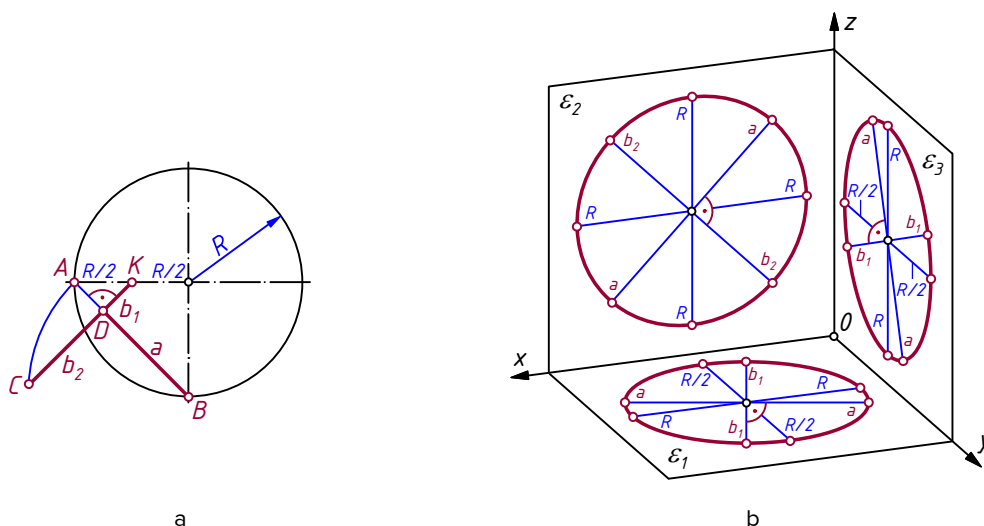
Joonis 3.91. Ringjoonte tuletamine standardses ristdimeetrias: a – pooltelgede tuletamine; b – koordinaatpindadel asetsevate ringjoonte kujutisellipsid.
