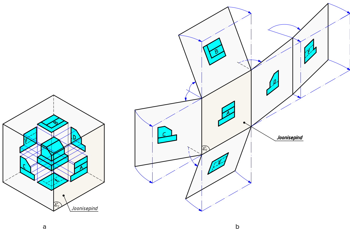
Joonis 4.5. Projekteerimine kolmanda ruuminurga meetodil.
