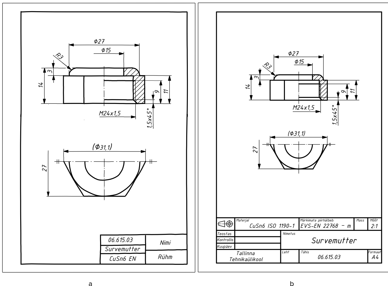
Joonis 4.175. Survemutri eskiis (a); tööjoonis (b).
