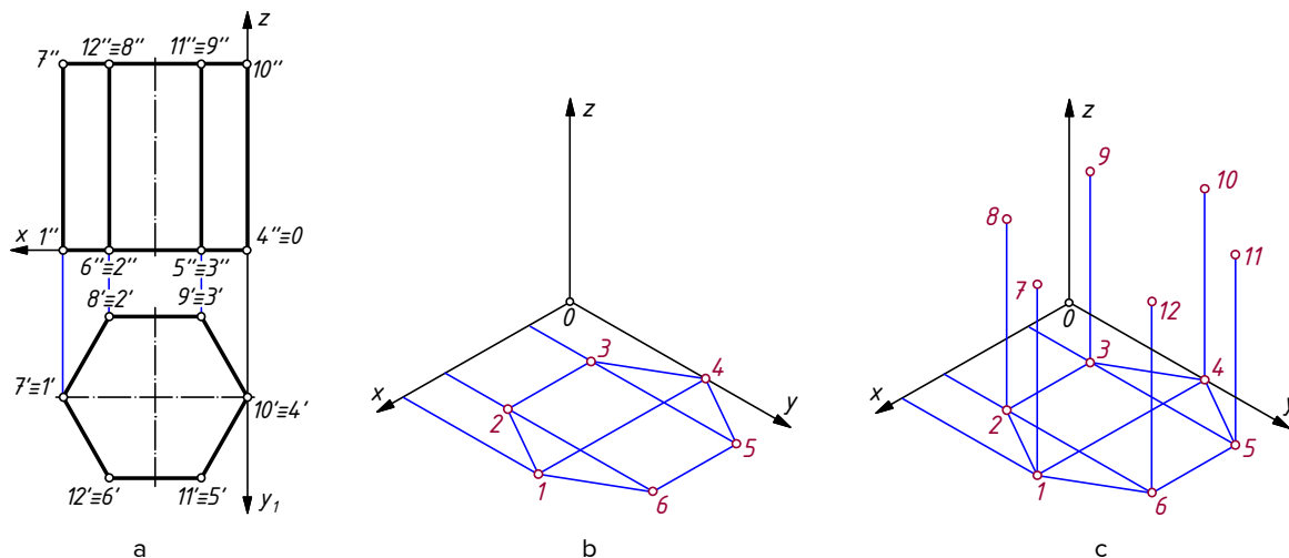
Joonis 3.105. Prisma aksonomeetrilise kujutise tuletamine: a – kaksvaade; b, c, d – tuletamine; e – tuletatud aksonomeetriline kujutis.
