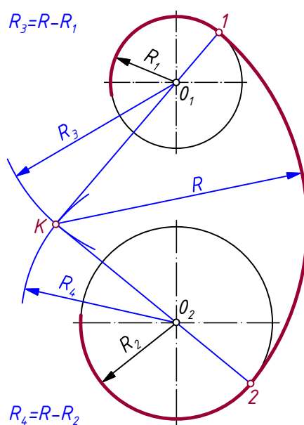
Joonis 2.22. Lookühend.
