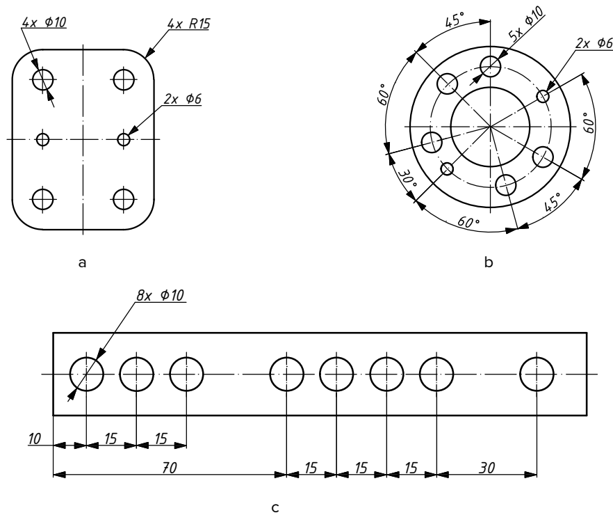
Joonis 4.97. Ebahühtlaselt asetsevate korduvate elementide mõõtmestamine.
