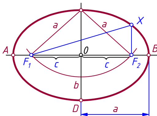
Joonis 3.126. Ellips.
