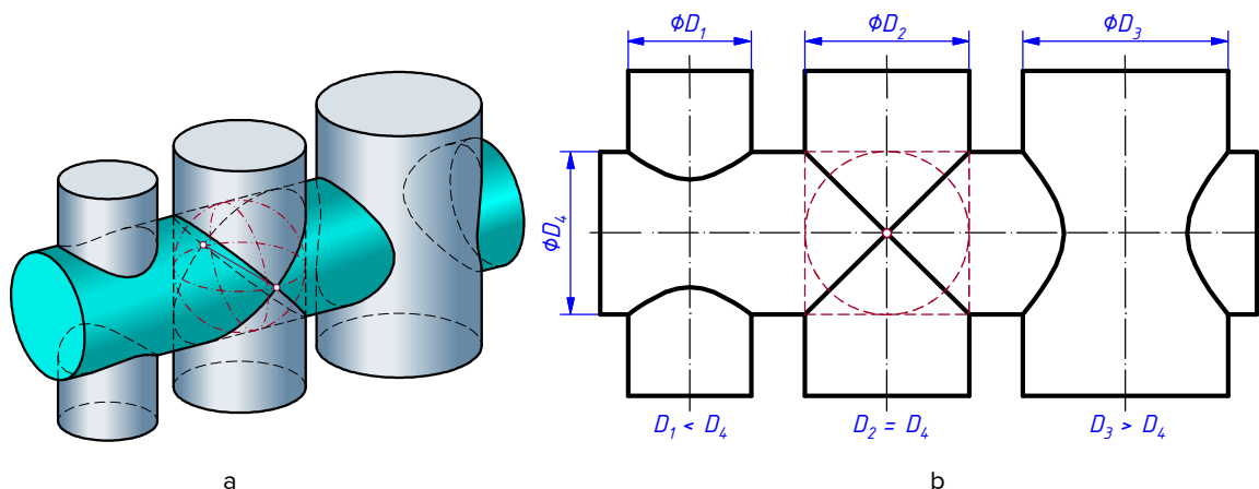
Joonis 3.189. Erinevate läbimõõtudega silindrite lõikumine: a – piltkujutis; b – eestvaade.
