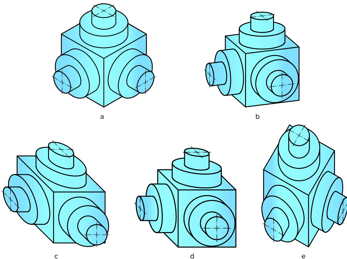
Joonis 3.95. Objekti kujutised aksonomeetrias: a – ristisomeetria; b – ristsdimeetria; c – frontaalne kalddimeetria; d – frontaalne kaldisomeetria; e – horisontaalne kaldisomeetria.
