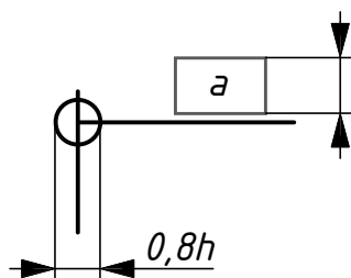
Joonis 4.64. Ühisnullpunkt.
