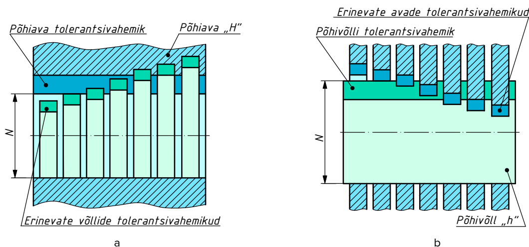
Joonis 4.150. Istude süsteemid: a – avasüsteem; b – völli süsteem.
