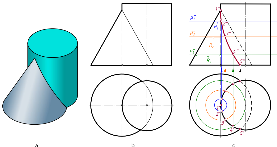
Joonis 3.184. Koonuse lõikumine silindriga: a – piltkujutis; b – lähteandmed; c – lahendus.
