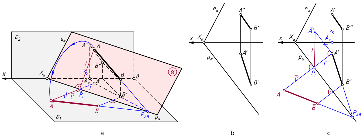
Joonis 3.77. Tasandi pööramine ümber põhijälje põhiekraanile: a – piltkujutis; b – lähteandmed; c – lahendus kaksvaatel.
