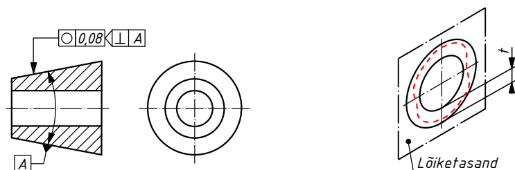
Joonis 4.159. Ümaruse tähistamine joonisel.
