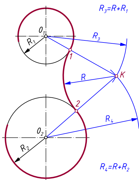
Joonis 2.21. Käändühend.
