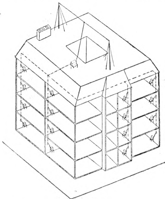
Joon. 1: Ühisvastuvõtuseadeldise skeem.
