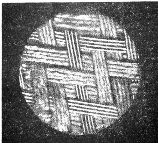
Joon. 2: Mikroskoopiline ülesvõtte segamiste vastu kaitstud antenni kudest.
