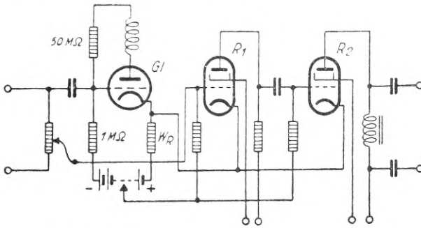
Joon. 1. Saatja juures kasutatav lülitis amplituudi kokkusurumiseks — „kompressor“.
