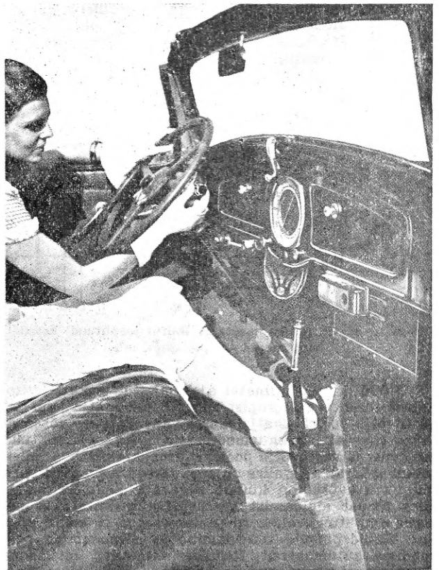
Raadiovastuvõtja paigutus autosse (Philipsi konstruktsioon). Juhuruumi esikülje all on näha vastuvõtja (paremal) ja valjuhääldaja (vas.). Rooliratta juurde on toodud häälestusnupud.
