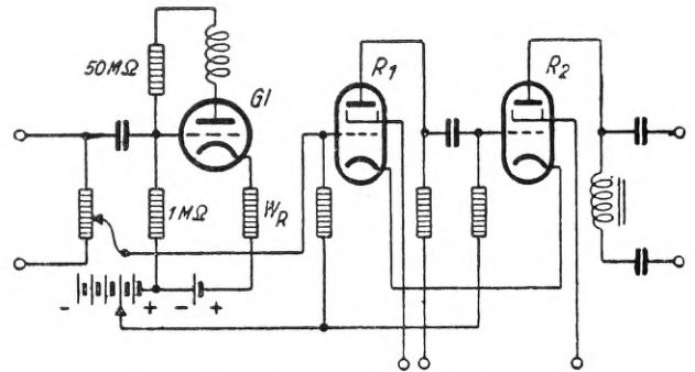
Joon. 2. Vastuvõtjas kasutatava „ekspanderi“ lülitis.
