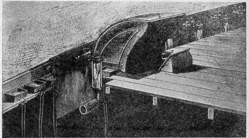
Ooperi ülekanDmine Pariisi ooperist 1881. Lava äärel, mis osalt kujutatud läbilõikes, on näha mikrofonid, mis gaasilampidest eraldatud vaheseinaga.
