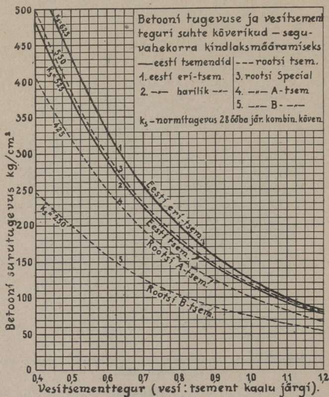
Joon. 9. Diagramm, mis näitab vahekorra betooni vastupidavuse ja vesitsemenditeguri vahel 28 ööbase kõvenemisaja järele. (A. G.)
