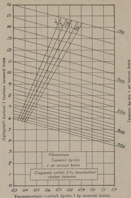
Joon. 30. Vahekord tsemendihulga, seguvahekordade ja vesitsementteguri vahel vibrobetooni jaoks.
