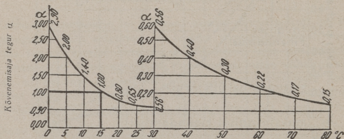
Joon. 4. Betooni kõvenemisaja sõltuvus temperatuurist. (A. G.)
