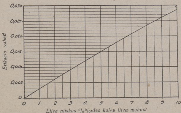
Joon. 14. Graafik, mis näitab „liiva niiskuse % kuiva liiva mahust“, olevalt „denaturaatpiirituse erikaalu vahest“.
