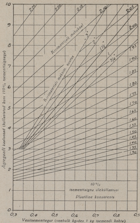
Joon. 26. Graafik plastilise betooni jaoks 10% tsementtaigna üleküllastusega.
