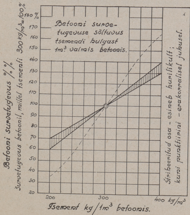
Joon. 1. Betooni tugevuse sõltuvus tsemendi hulgast 1 m 3 valmisbetoonis plastilise konsistenti puhul (Hummuli järgi). (A. G.)
