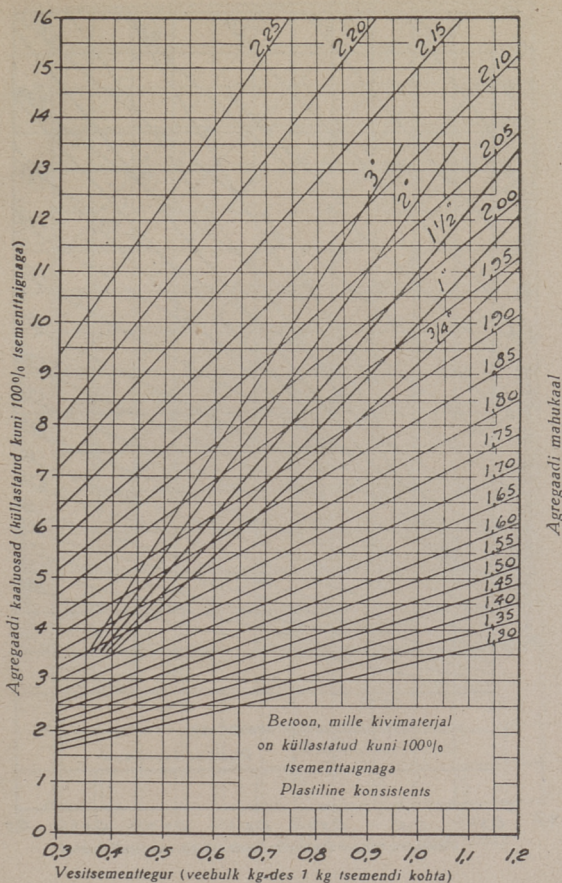
Joon. 25. Graafik plastilise betooni jaoks, milles õõnsused 100% ulatuses on täidetud tsementtaignaga.
