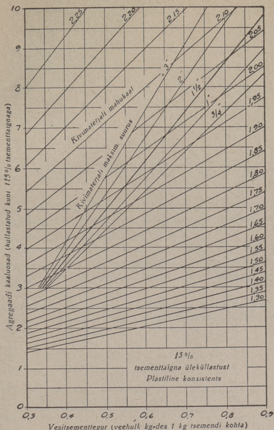
Joon. 27. Graafik plastilise betooni jaoks 15% tsementaigna üleküllastusega.
