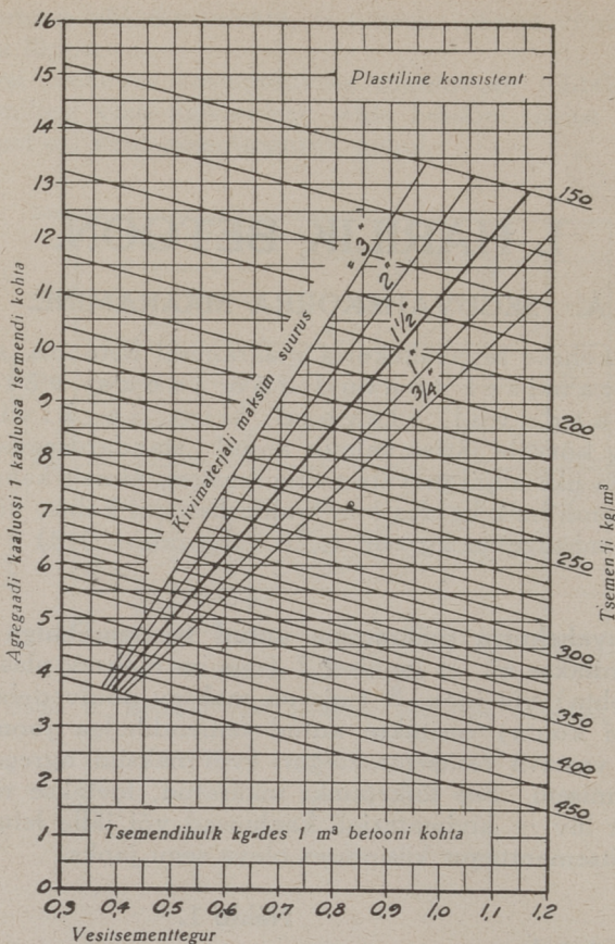
Joon. 7. Seguvahekorra määramise diagramm plastilise konsistentsiga betooni jaoks.
