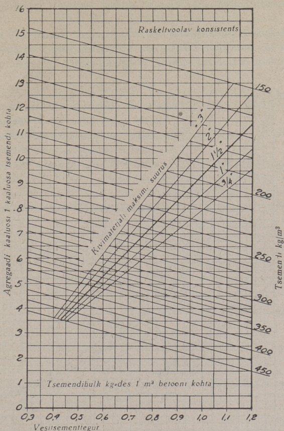
Joon. 8. Seguvahekorra määramise diagramm raskeltvoolava konsistentsiga betooni jaoks.
