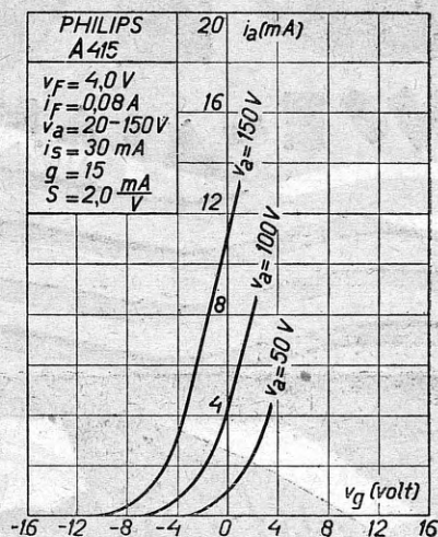
Philips audion, madalsagedus- kõvendajalamp A 415
