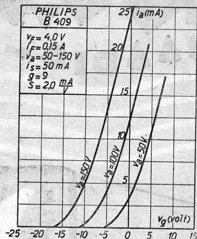
Philips lõpukõvendaja, madal- sageduskõvendajalamp B 409
