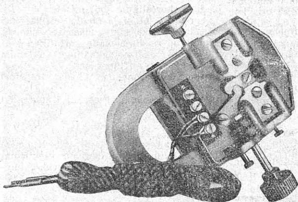
„Isophoni“ moodne ümberlülitav magnet-süsteem
