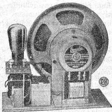
„Excello-Domo“ dünaamilise väljuhääldaja shassii ühes väljumise trafo ja lampaladajaga
