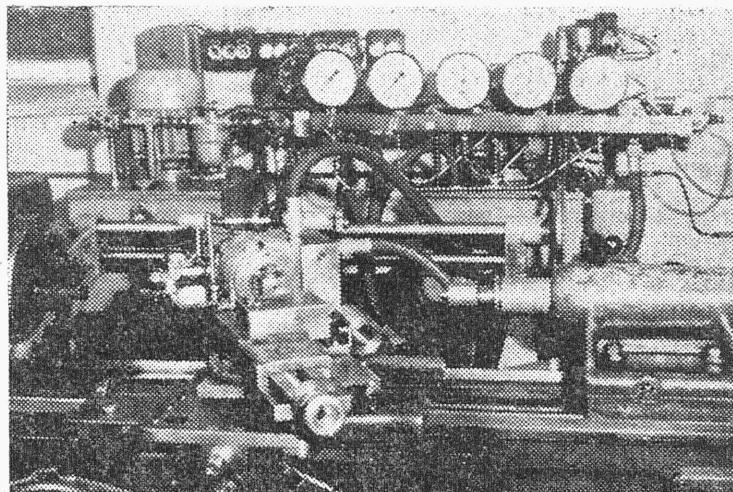
Masinaehit. tehn. kat. Hüdrokopeerisupportide katsetamise stend.
