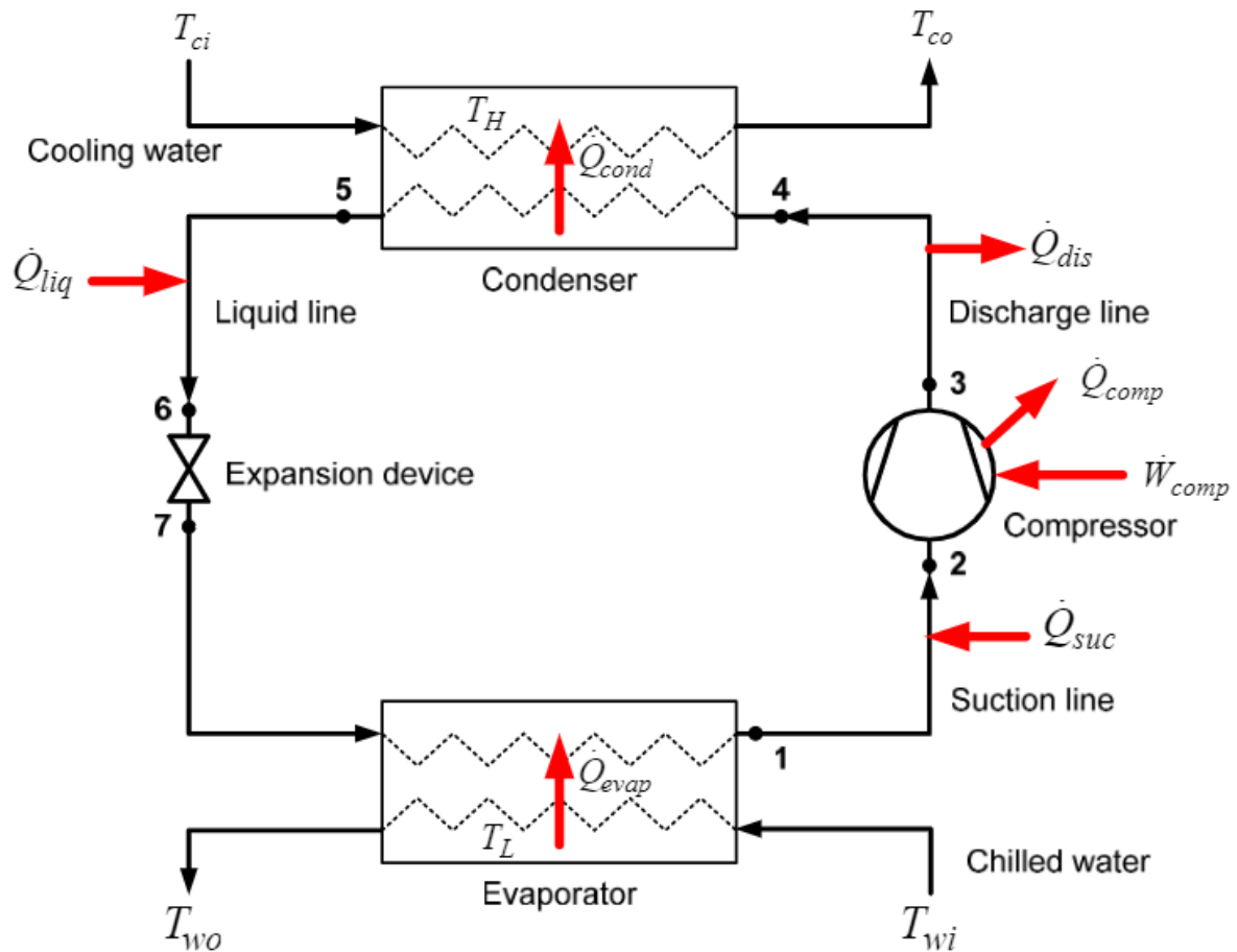
Joonis 2.2. Kompressorjahuti põhimõtteline skeem
