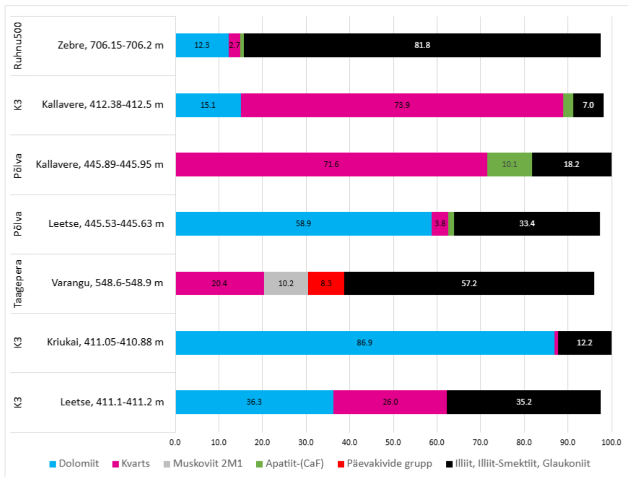
Joonis 29. Lõuna-Eesti puuraukude proovide AU24-11–AU24-17 mineraalne koostis XRD analüüsi põhjal. Joonisel on kujutatud mineraalid, mis moodustavad üle 5%, mittekvantifitseeritud väärtused sisaldavad endas illiiti, illiit-smektiiti ja glaukoniiti.
