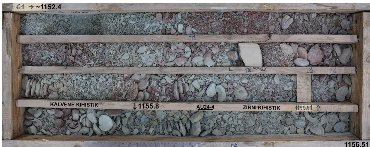
Kast 61. Zirni kihistiku hallikas savi, sügavusel 1155.8 ilmuvad esimesed Kalvene punakas hallid mudakivid. Esinevad esimesed paksemad karbonaatsed vahekihid. AU24-4 võetud sügavusel 1156.1 m.
