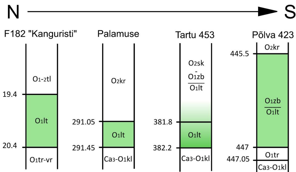
Joonis 33. Leetse kihistu põhja-lõuna suunaline profiil, Tartu 453 ja Põlva 423 läbilõikes on Zebre kihistu loetud Leetse kihistuks. F182 puursüdamik on joonistatud Puura jt (1977) andmete põhjal. Palamuse läbilõige on joonistatud Kõrvel jt (1963) andmete põhjal.
