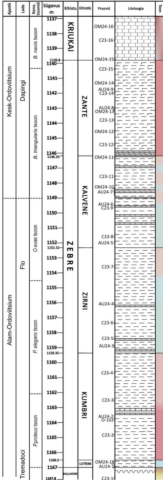
Joonis 31. Aizpute-41 läbilõige Liefroy (2024; personaalne kommunikatsioon, 2026) esmase biostratigraafilise analüüsi andmetel.
