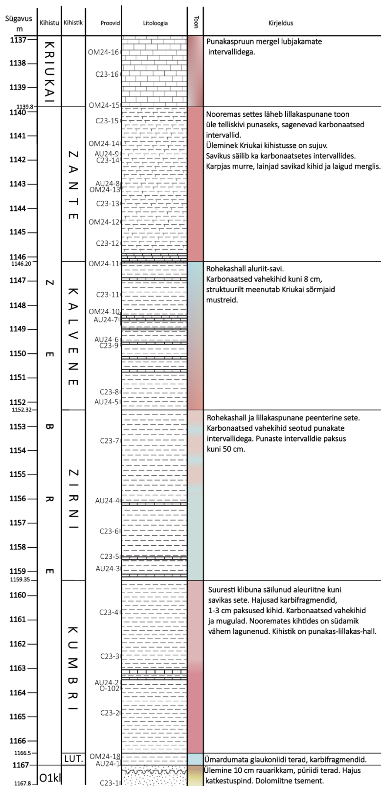
Joonis 11. Aizpute puursüdamiku litoloogiline läbilõige koos lühikirjeldusega.
