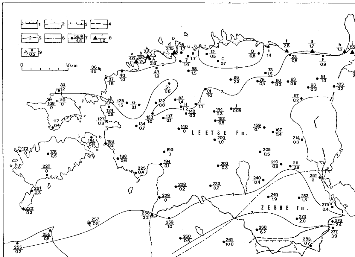
Joonis 8. Hunnebergi ja Billigeni lademe levik Eestis. Joonisel on näha täpitatud punktiirjoonega märgitud teoreetilist Zebre kihistu levikut. 258 – Ikla, 249 – Otepää, 253 – Põlva, 273 – Võru, 275 – Värska, 276 – Petseri, 283 – Hino (ei ole säilinud), 268 – Karula, 269 – Laanemetsa (ei ole säilinud). Kihipaksuste andmed pärinevad Rõõmusoks (1960), Orviku (1960a), Männil (1966), Rõõmusoks (1983) ja L. Põlma avaldamata andmetel. Zebre kihistu leviku piir on joonistatud Ulst (1982) kaardi järgi Meidla (1997a) poolt.
