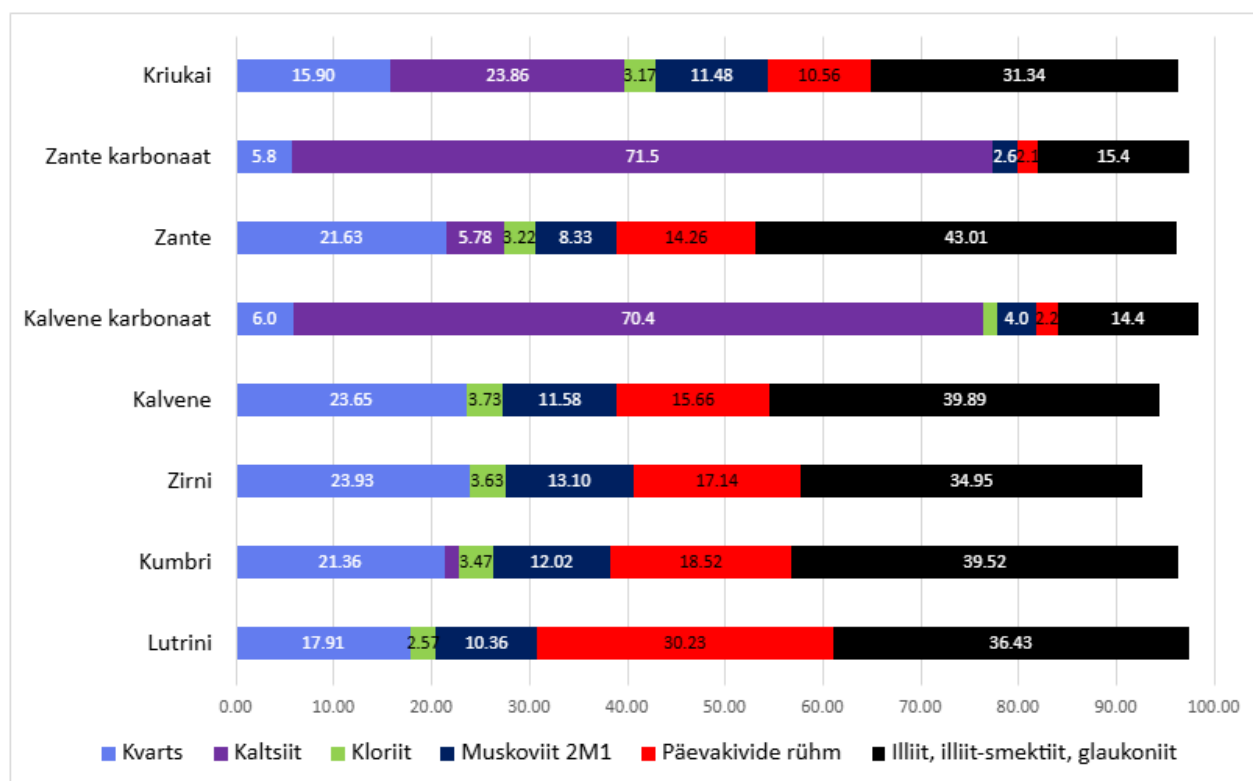
Joonis 14. Zebre kihistike keskmistatud mineraalne koostis XRD tulemuste järgi (lisa 3). Mineraalide loetelust on välja arvestatud apatiit, jarosiit, kips ja dolomiit – nende sisaldus oli alla arvestust. Kihistikud/kihistud on reastatud alt-üles vanemast nooremani.
