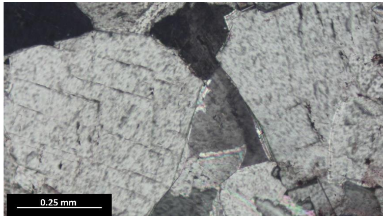
Joonis 22. Kuressaare K3 puuraugu proovi AU24-12 (411.05–410.88 m, Kriukai kihistu) õhik. Dolomiidikristallid polariseeritud valguses.
