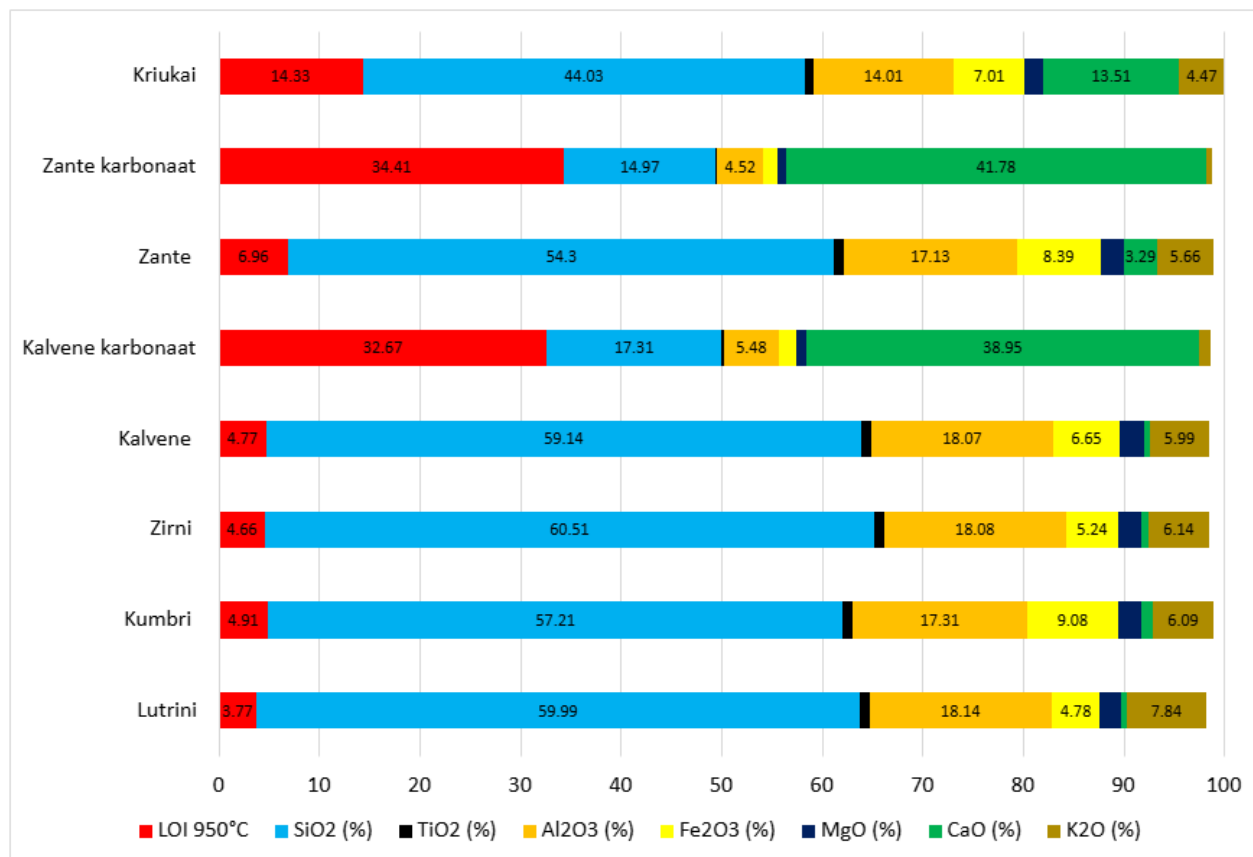
Joonis 15. Zebre kihistike makroelementkoostis, graafikul on kujutatud savikate intervallide keskmistatud väärtused kihistiku kaupa XRF sulatusmeetodil (lisa 2). Kihistikud on keskmistatud arvestamata karbonaatseid proove.
