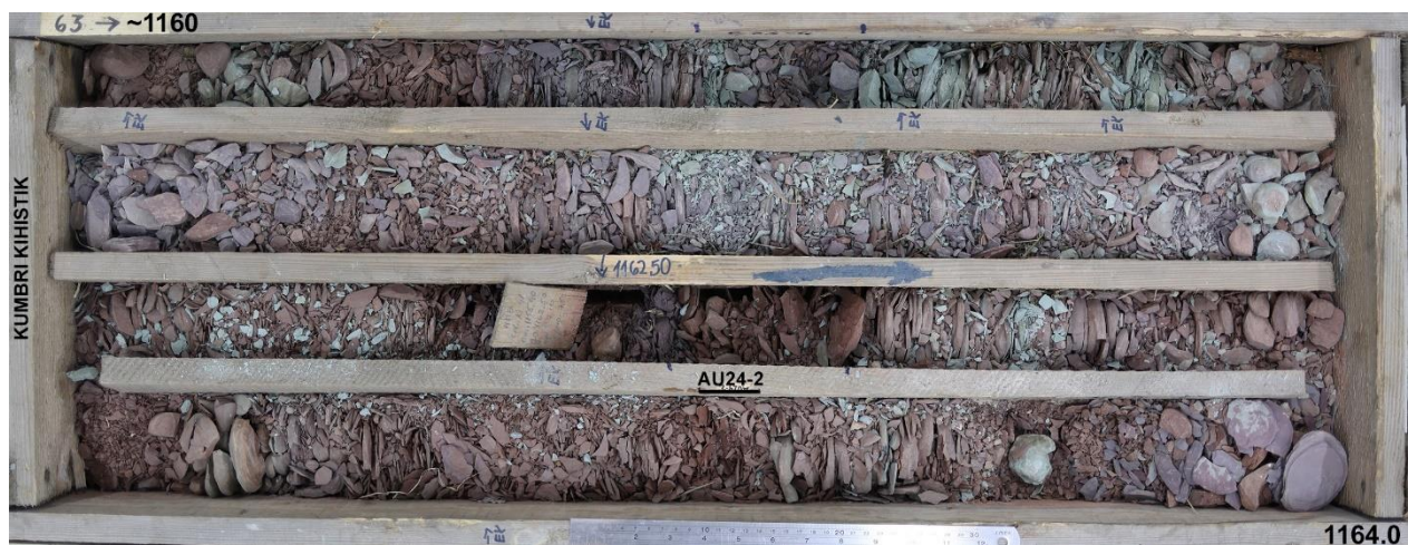
Kast 63. Kast sisaldab Kumbri kihistike punakat setet. Hall lisand on pudenenud teisest kastist. Proov AU24-2 on sügavusel 1163.57–1163.62.
