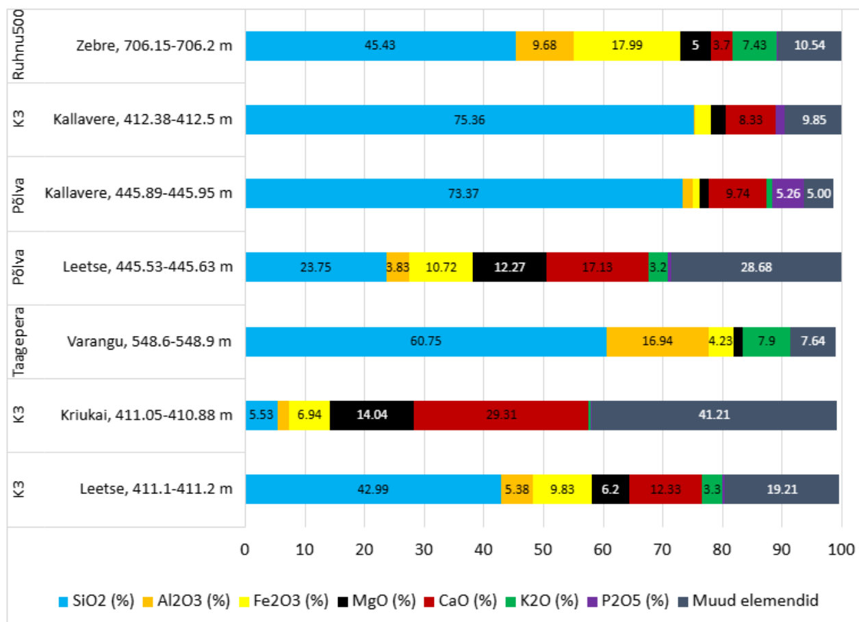
Joonis 28. Lõuna-Eesti proovide geokeemia XRF sulatusmeetodil. Muud elemendid on CO 2 , TiO 2 , MnO, Na 2 O, SO 3 ja Cl.
