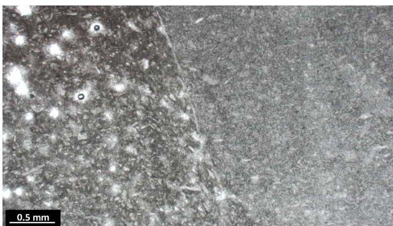
Joonis 13. Aizpute-41 puuraugu proovi AU24-9 õhik, jäljekivistise täite külgprofiil selgelt eristatava terasuuruse erinevusega. Jämedateraline pool on hiljem täitunud.
