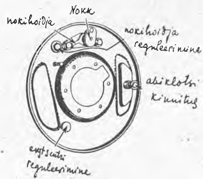
Pilt 11. Bendix-piduriseade reguleerimine.
