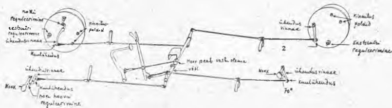
Pilt 10. Essex 1928. a. tüüpi Bendix-piduriseade skeem.
