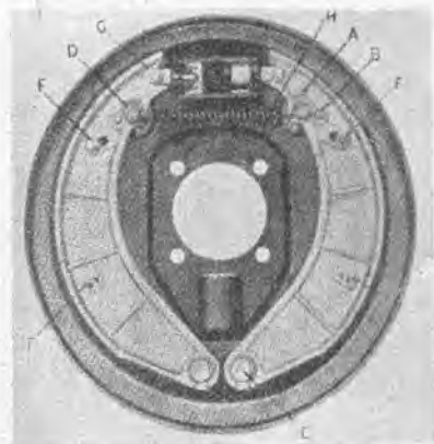
Pilt 8. Lockheed-piduri klotside asend.
