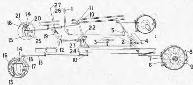
Pilt 6. Oldsmobile 1928. a. tüüpi pidurite skeem.
