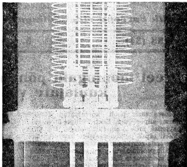
Röntgeniülesvõte Philipsi suursaate-lambi anoodi ülemisest osast ühes võre ja kütetraatidega.
