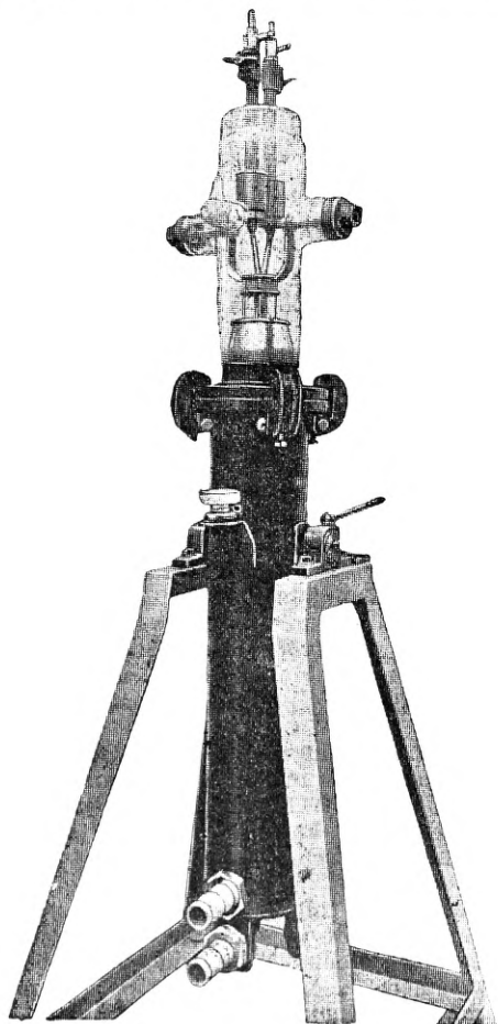
Philipsi 350-kW-ne hiigellamp.
