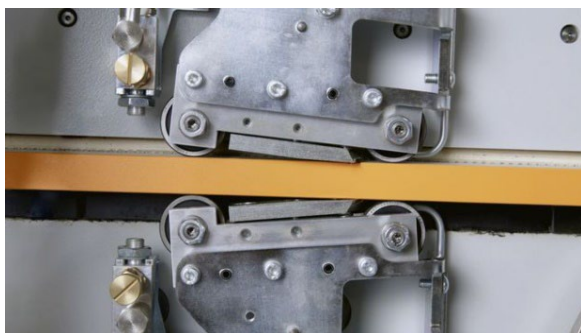
Joonis 6.21 Liimieemaldusnood ja puhastusrullid. Foto: HOLZ-HER GmbH
