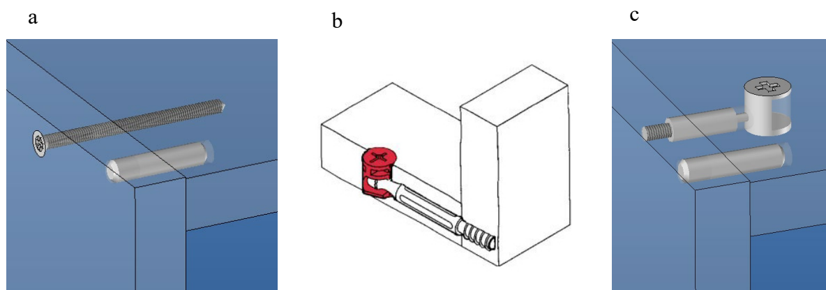
Joonis. 9.17 Korpasmööbli seotistes kasutatavad tõmmitsad: a – tüübel ja koostekruvi, b – ekstsentriskõmmits, c – tüübel ja ekstsentriskõmmits.
