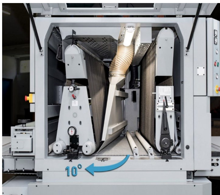
Joonis 1.100 Kontaktvaltsi ja surveelemediga lailintlihvping (surveelement on etteande suhtes ristasendist pööratud). Foto: Kündig AG
