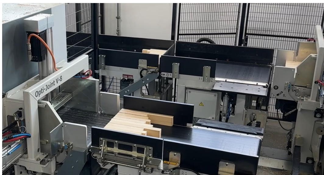
Joonis 4.21 Vertikaalsõrmtapi freesimis- ja liimitamisseade. Foto: S. Kooli
