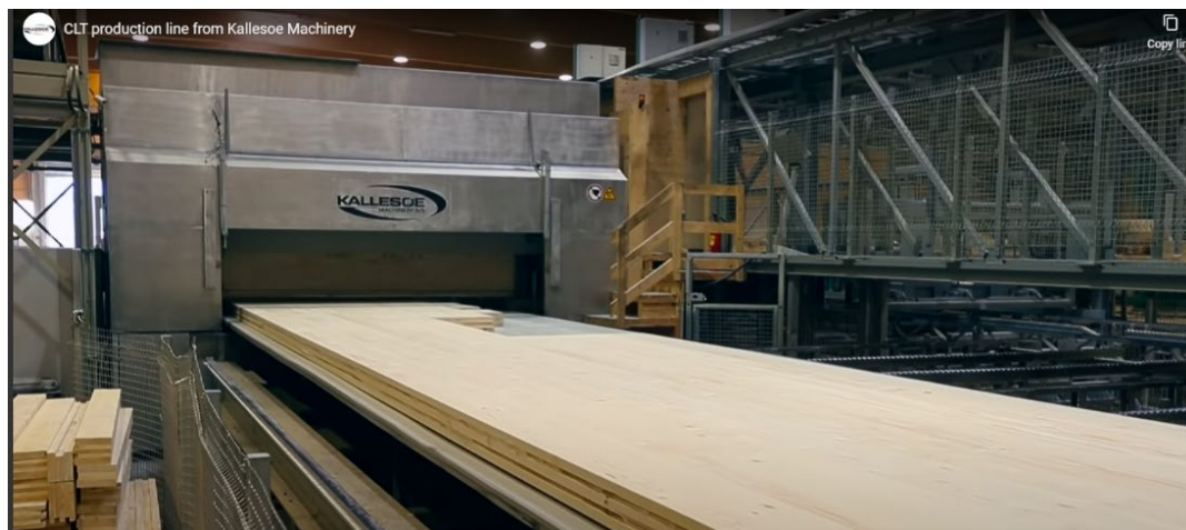
Joonis 10.60 Hasslacher Norica Timber ja kõrgsageduspressi tootja Kallesoe kulusäästlik ristkihtliimpuitpaneelide pressimisliin, kus avadesse puitu ei panda.
