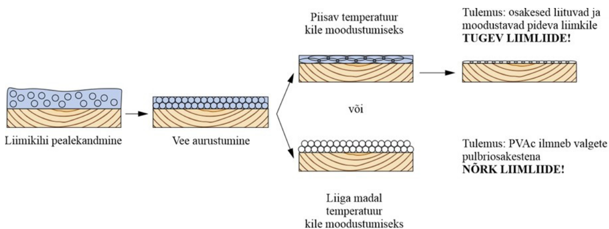
Joonis 5.5 PVAc liimikile moodustumine ja kõvenemine liiga madalal ja piisaval temperatuuril.
