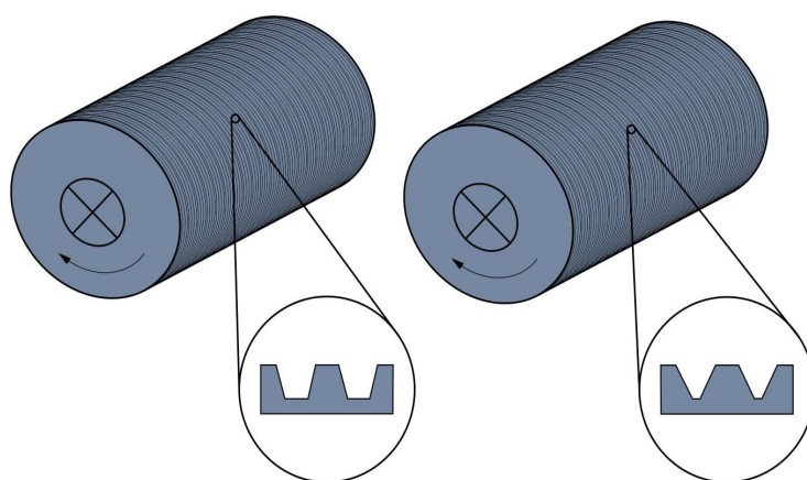
Joonis 5.11 Liimivaltside soonte profiilid.
