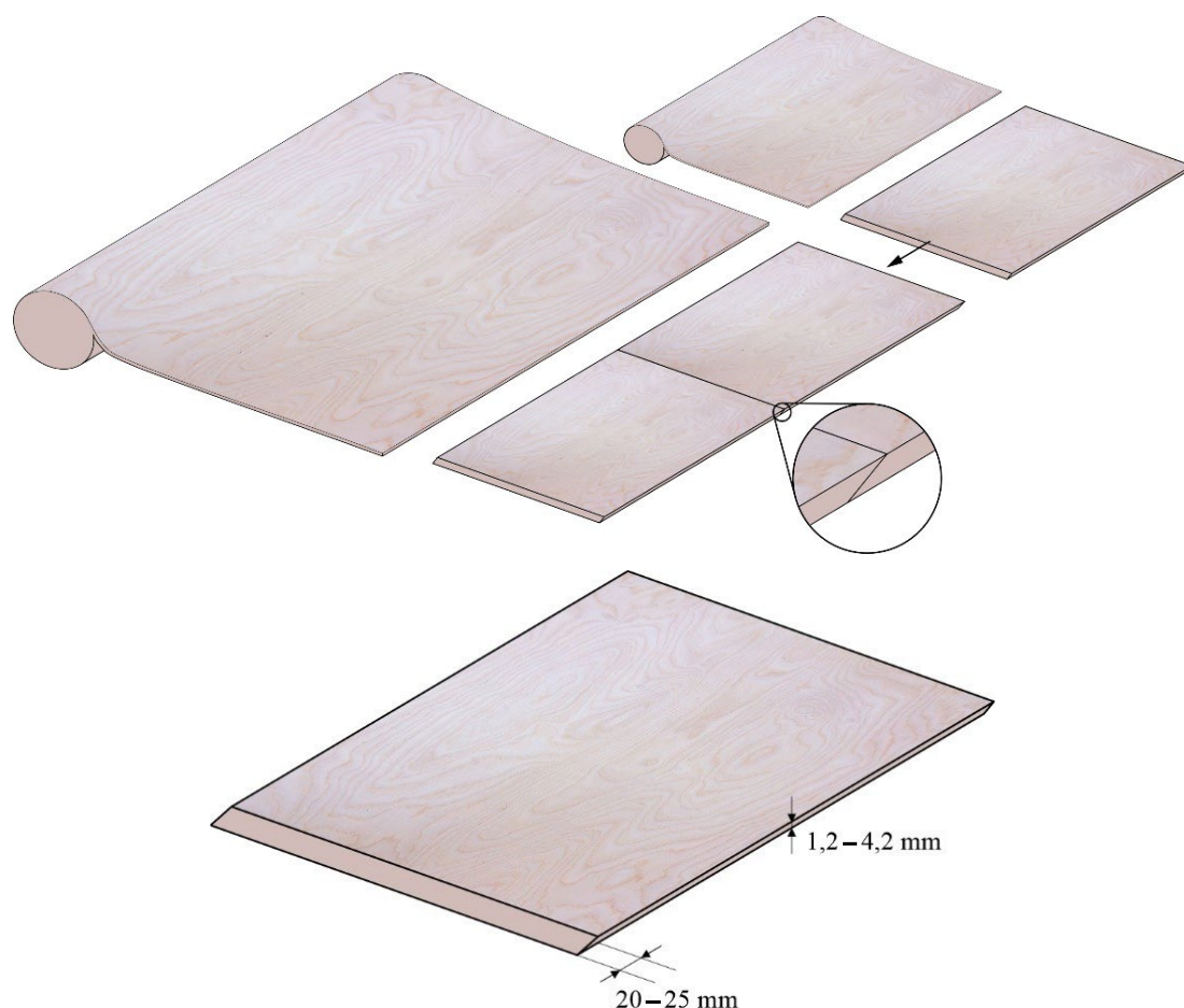
Joonis 5.53 Pikijätkamise spoon ja pikijätku mõõtmed.
