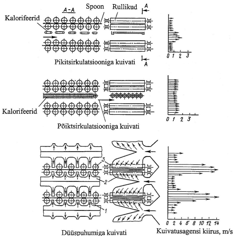
Joonis 3.33 Rullkuivatite tüübid: 1 – dүүsid, 2 – tsirkulatsioonikanalid, 3 – rullikud. Joonis: R. Reiska
