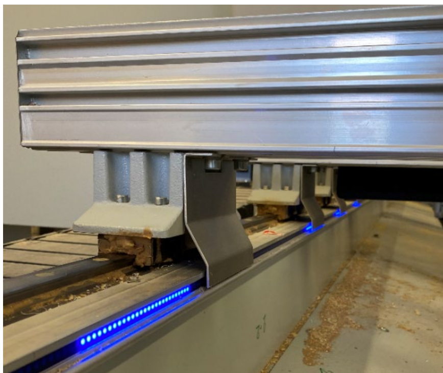
Joonis 7.37 Töötlusprogrammile sobiv vaakumkonsooli asetus (asukohad on operaatori töö hõlbustamiseks näidatud LED-tuledega).
