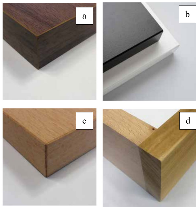
Joonis 6.9 Servapealistused: a – melamiin, b – PVC/ABS, PP, c – ribastatud spoon, d – krepp ehk täispuit. Foto: SCM Group
