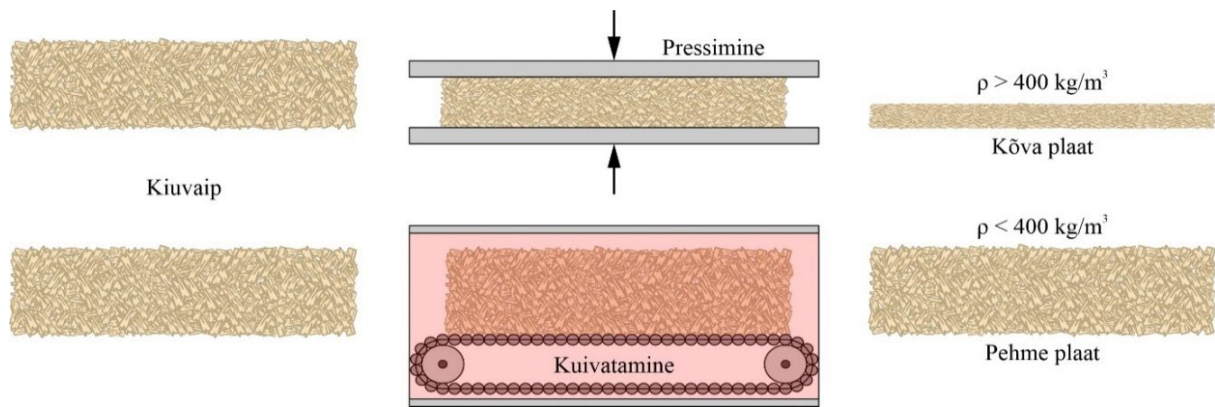
Joonis 5.94. Märgmeetodil kõvade ja pehmete puitkiudplaatide valmistamine.
