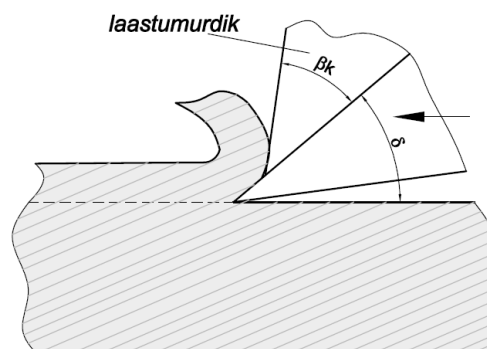
Joonis 1.25 Laastu moodustumine pikilõikamisel laastumurdiku kasutamisel.
