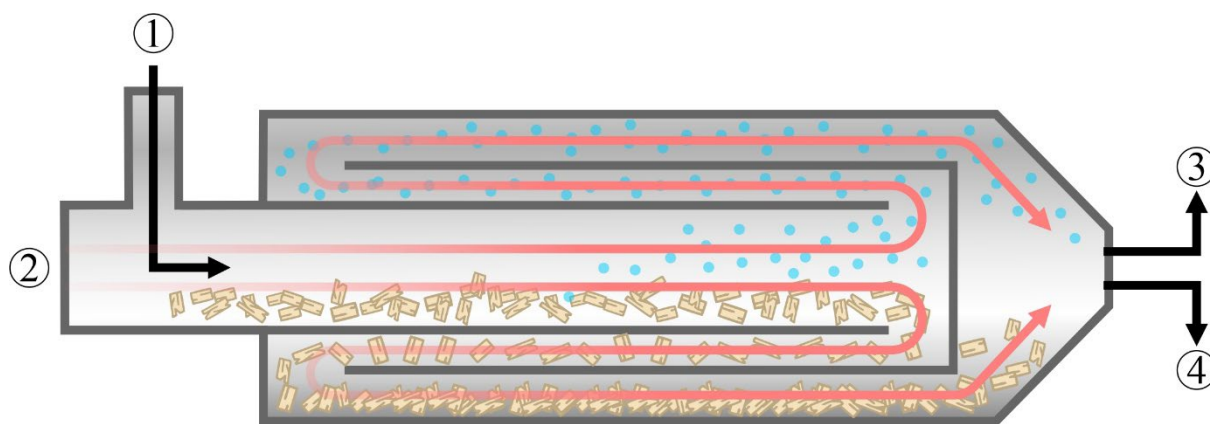
Joonis 3.49 Kolmekäiguline Bizoni trummelkuivati: 1 – toitesead, 2 – küttekolle, 3 – gaasikäik kuivatusagensi retsirkulatiooni; 4 – kuivatatud laast välja.
