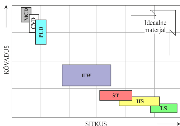
Joonis 1.29 Erinevate materjalide kõvadus- ja sitkusnäitajad: MCD – monokristalliline teemant, CVD – aurufaasist keemiliselt sadestamisel saadud polükristalliline teemant, PCD – polükristalliline teemant, HW – kõvasulam, ST – stelliit, HS – kiirlõiketeras, LS – legeerteras.
