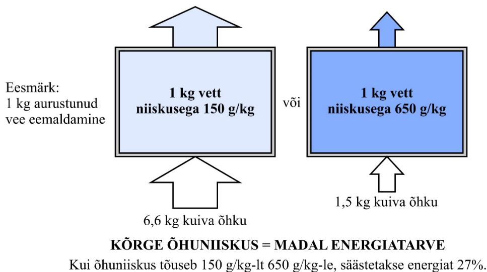
Joonis 3.42 Spoonikuivati õhuniiskuse mõju energiatarbele.
