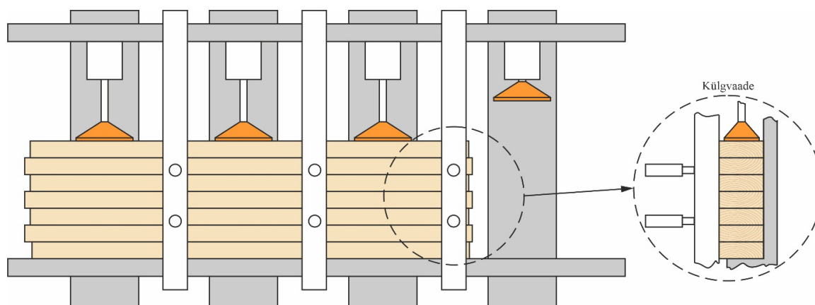
Joonis 5.15 Seinpress.
