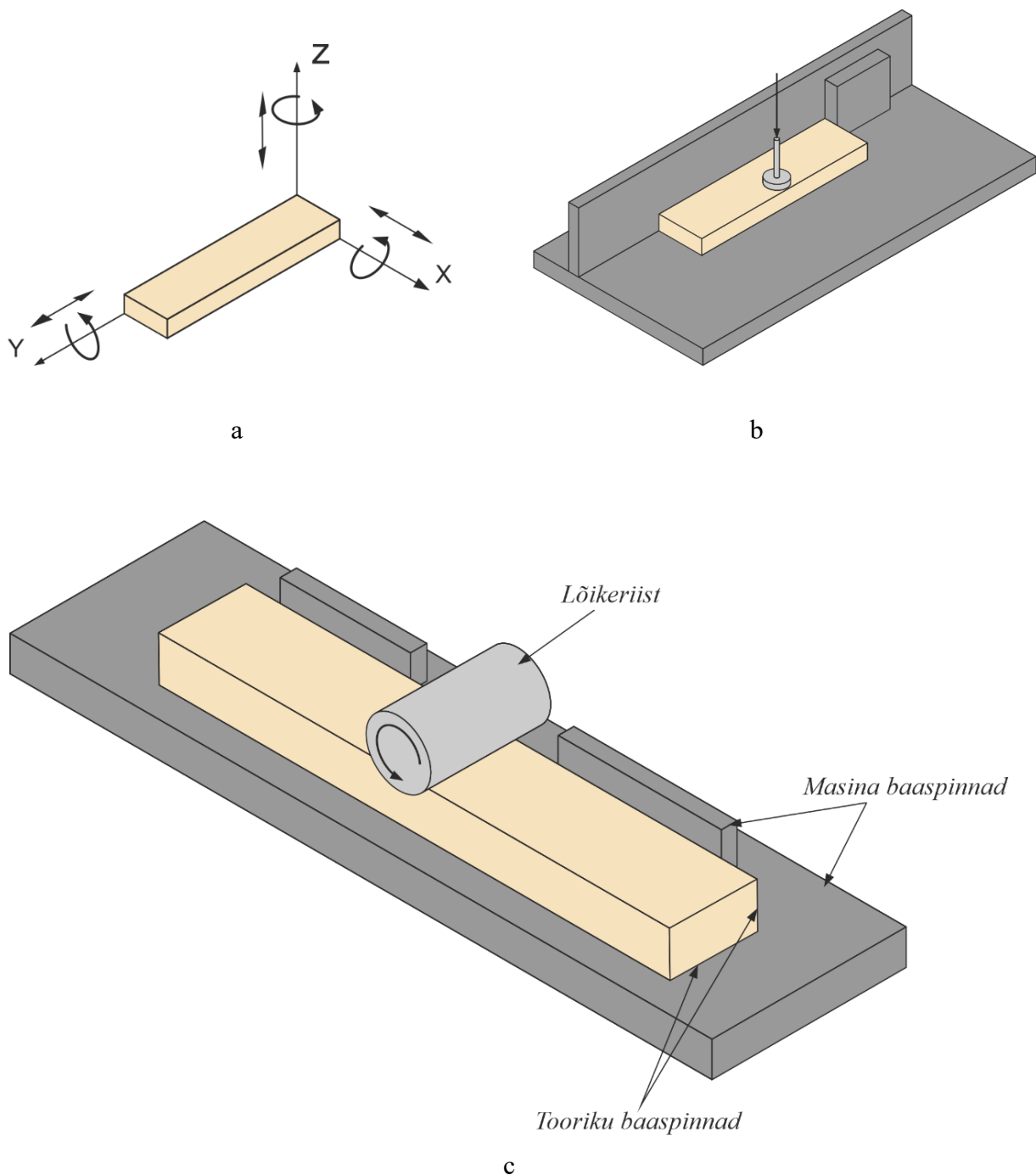
Joonis 4.6 Baaspinnad puitdetailide töötlusel: a – keha kuus vabadusastet ruumis, b – liikumatu baseerimine, c – liikuv baseerimine.
