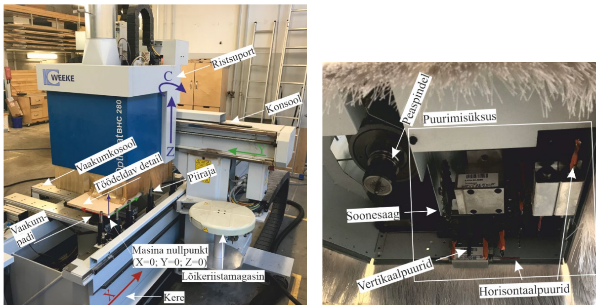
Joonis 7.1 3+1-teljeline Weeke CNC-töötlemiskeskuse põhiosad. Joonis: K. Kiiman
