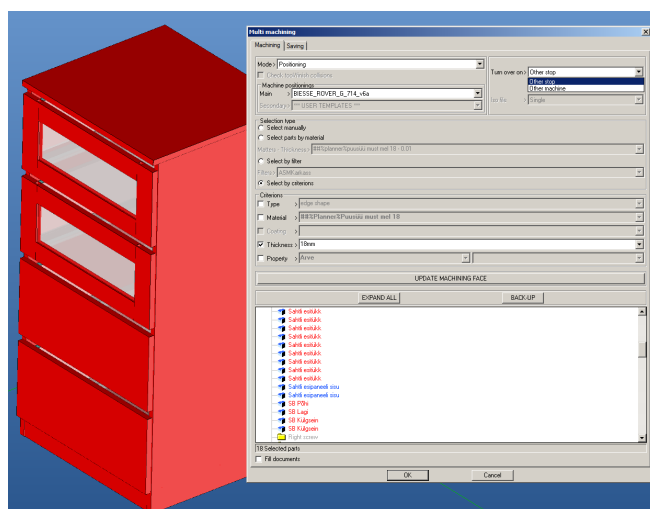
Joonis 10.44 Detailide lõiketöötlusfaili genereerimine CNC-pingile. Autor: M. Muru
