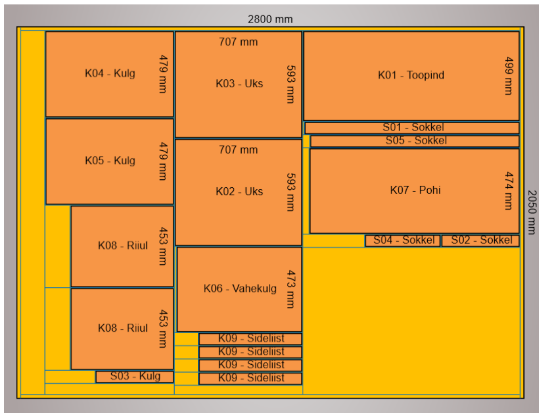
Joonis 6.7 Optimeeritud lahtilõikuskava kapi melamiinpladist detailidele (kasutatud MaxCut vabavara). Joonis: K. Kiiman
