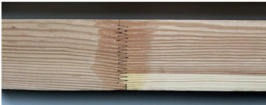
Joonis 4.31 Sõrmjätatud tooriku liimliite kontrollimine joodiga.
