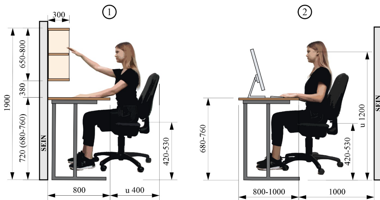
Joonis 9.1 Mõõtmed töötamisel: 1 – töölauda taga istudes, 2 – arvutiga töötamisel.
