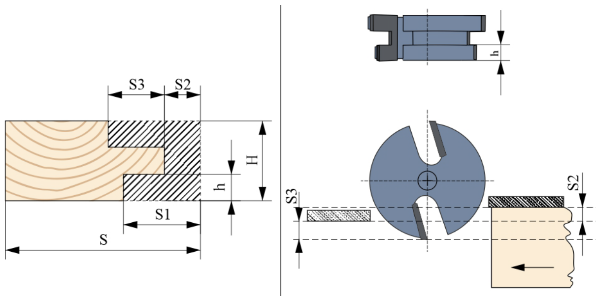
Joonis 1.70 Universaalfreesi juhtjoonlaudade paiknemine kujufreesimisel.
