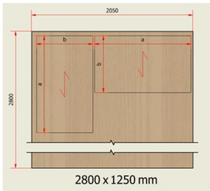
Joonis 6.6 Pikisüüsuunaga plaat koos piki- ja ristisüüsuunaga detailidega. Joonis: K. Kiiman
