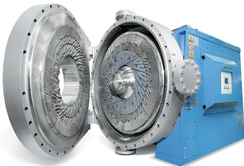
Joonis 5.84 Seade hakke järelopeenestamiseks. Foto: Audritz AG
