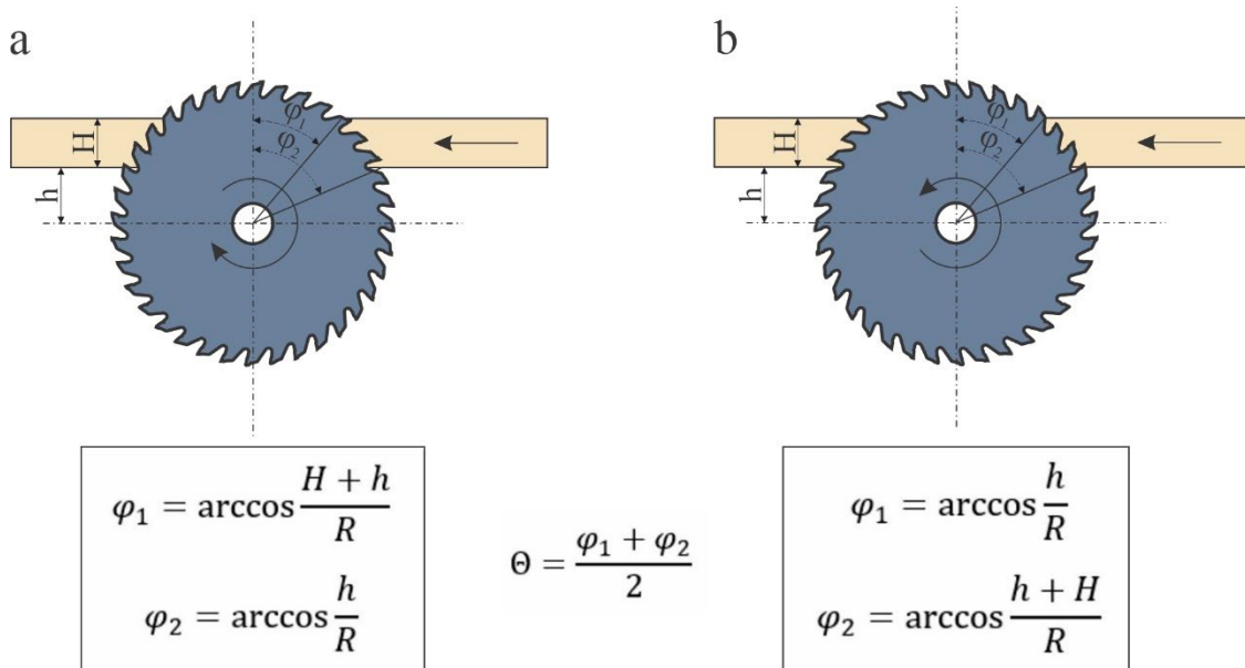
Joonis 1.36 Kinemaatilise kohtumisnurga leidmine, kui saag on töölaua all. Vasakul vastuetteanne, paremal pärietteanne.
