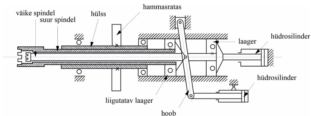
Joonis 1.91 Spoonitreipingi kaheosaline spindel.
