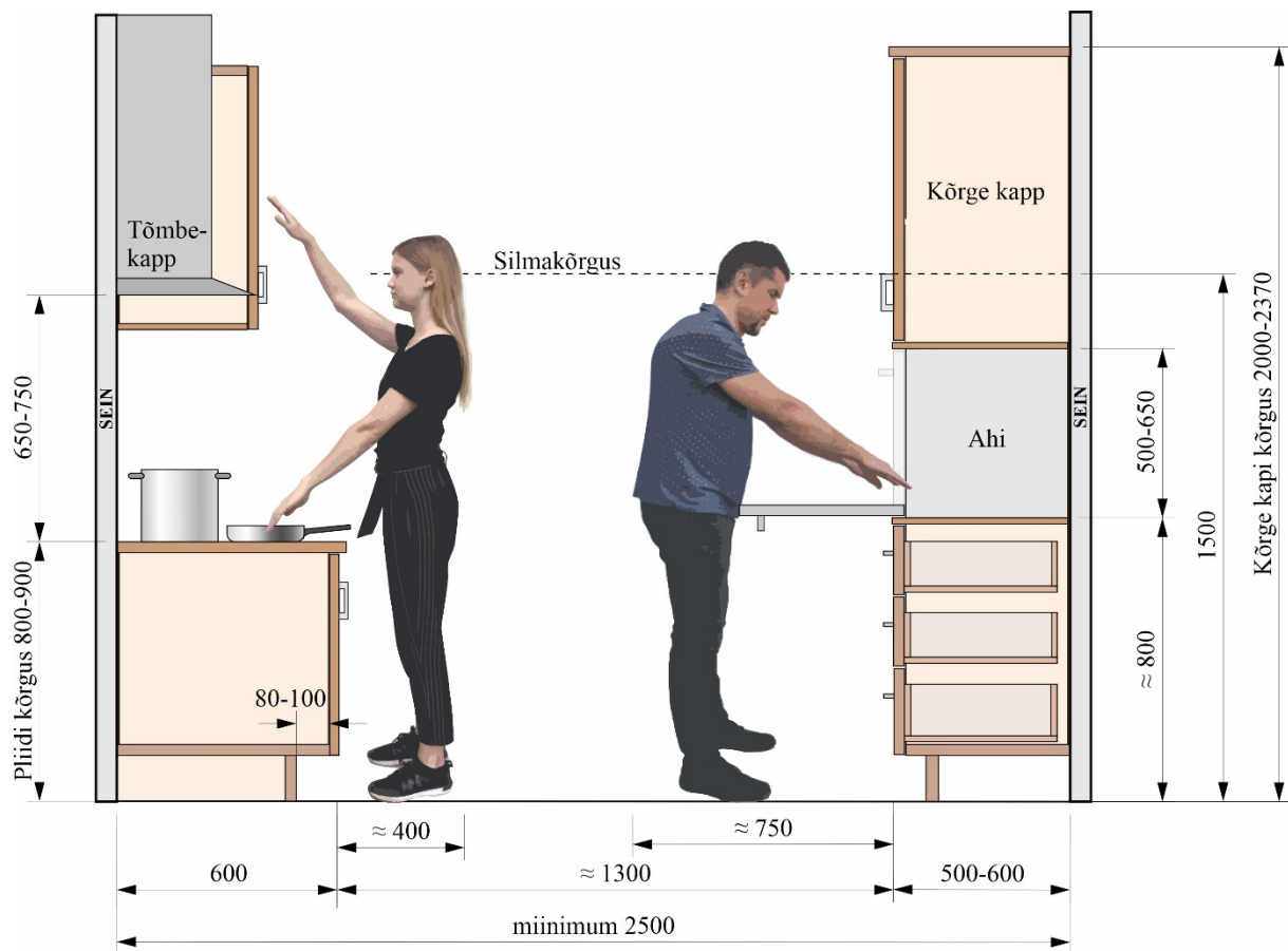
Joonis 9.3 Kööginõu mõõtmed köögitehnikaga töötamiseks.
