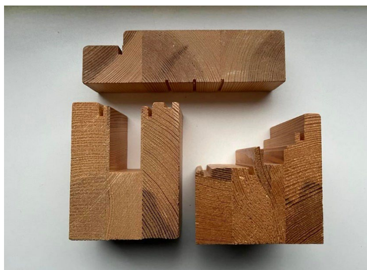
Joonis 4.30 Mitmest sõrmjätkatud lamellist aknaprofiili (all) ja ukسلengiprofiili (üleval) ristlõiked.
