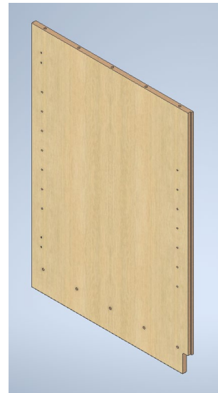
Joonis 7.26 Vertikaalne CNC-töötlemiskeskus ja näide võimalikust töödeldavast detailist. Foto: HOMAG Group AG. Joonis: K. Kiiman
