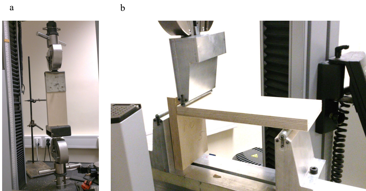
Joonis 9.35 Liidete tõmbe- ja nihkekatse: a – tõmmitsaga sileservliite katsetus tõmbele, b – T-kujulise tõmmitsaga nurkliite katsetus nihkele katseseadmél Instron 5866. Fotod: K. Saar
