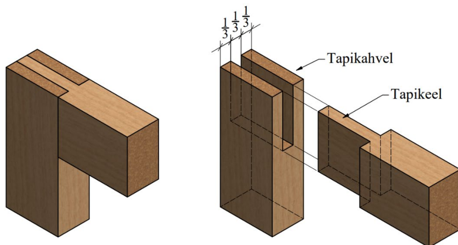
Joonis 9.43 Harktapi koostisosad: tapikahvel ja tapikeel, mille asend fikseeritakse liimiga.
