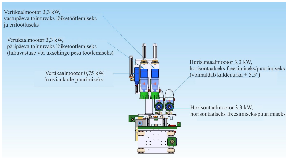
Joonis 7.48 CNC-pingi suurti konfiguratsioon lenglade läbisöötmiseks (teine suurti on samasugune, aga peegelpildis).
