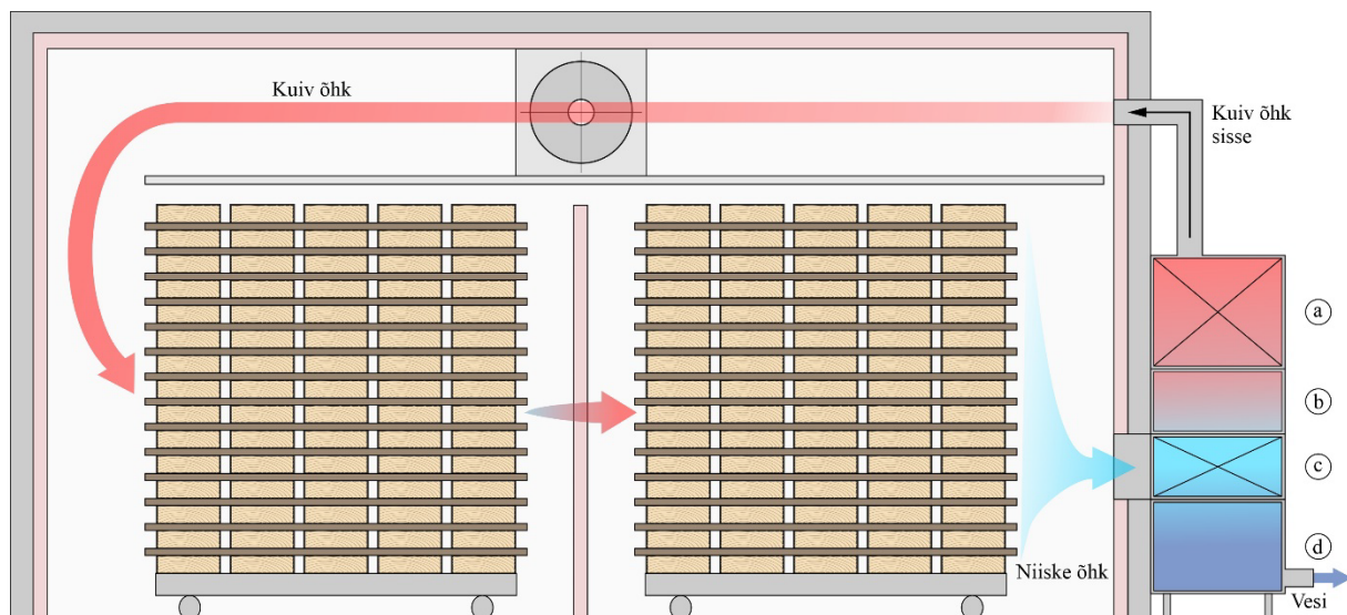
Joonis 3.23 Soojuspumbaga kondensatsioonkuivati tööpõhimõte: a – õhusoojendi kuivatusagensi soojendamiseks, b – kompressor, c – soojusvaheti – niiske ja sooja õhu sisseimamine ja mahajahutus, (d) – kondensaator – kondensvee väljund.
