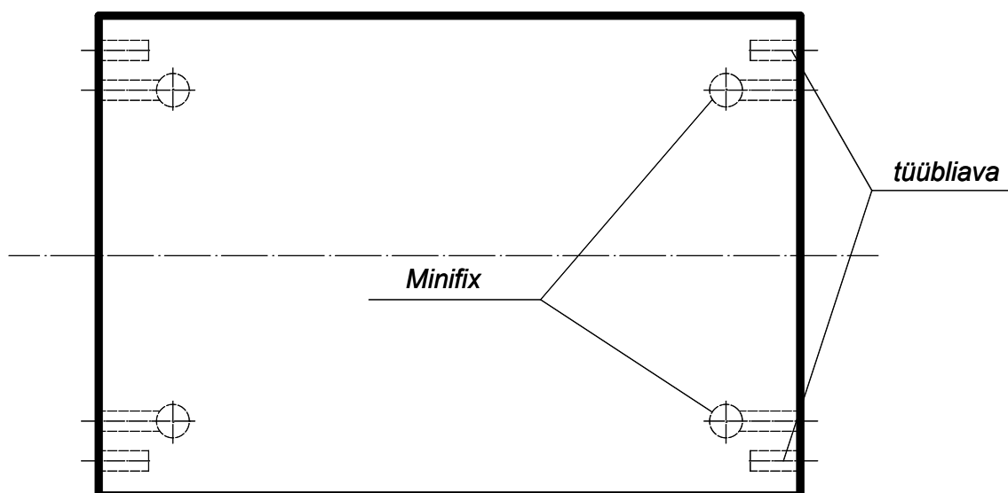
Joonis 9.19 Mööblidetail puittüüblite ja ekstsentriktõmmitsate jaoks puuritud avadega (kahe tüübli ja ühe ekstsentriktõmmitsaga liide pealtvaates).
