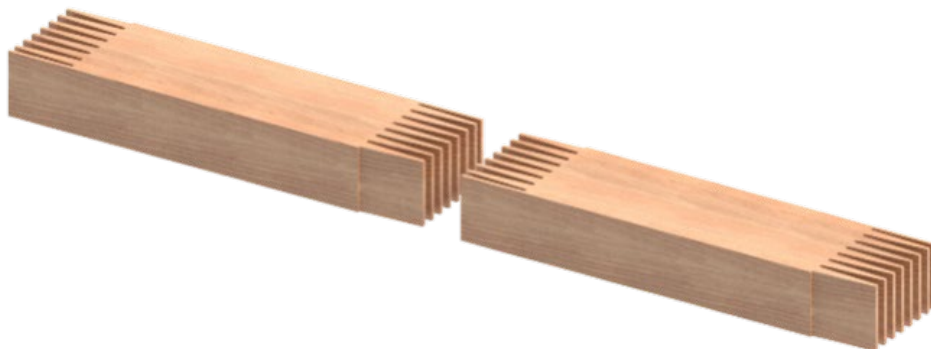
Joonis 4.19 Vertikaalsõrmtapp.
