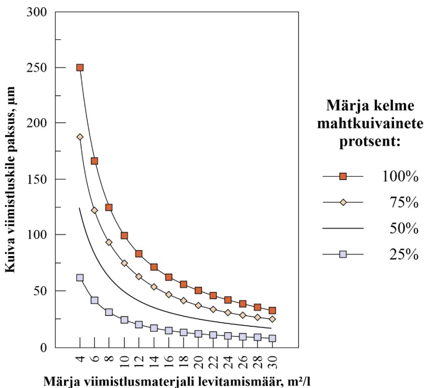
Joonis 8.19 Pinnale kantud märja viimistlusmaterjali kogusele vastav viimistluskile paksus.
