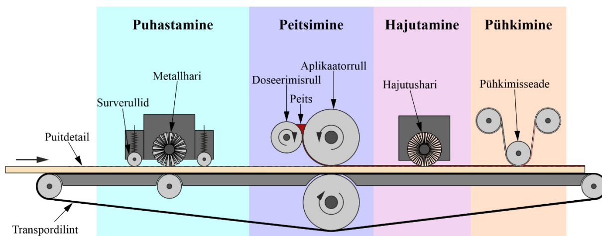
Joonis 8.13 Valtsirullidega peitsmasina põhimõtteskeem.
