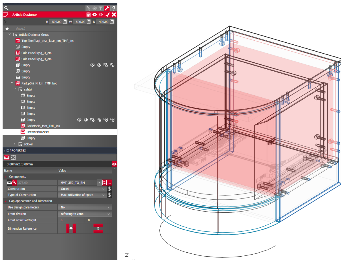
Joonis 10.7 Article Designer tööriistaga loodud sahtliga öökapi 3D-mudel. Autor: P. Nool
