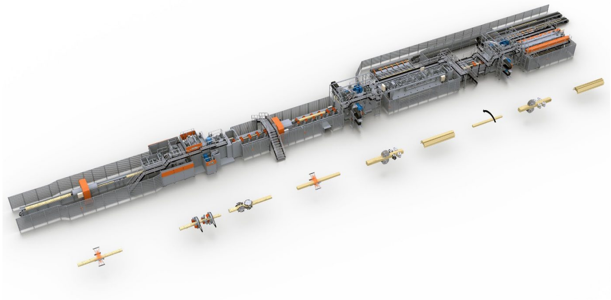
Joonis 2.40 Saeliin HewSaw SL250 3.3. Foto: Veisto OY
