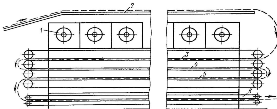
Joonis 3.38 Võrkkuivati põhimõtteskeem: 1 – telgventilaator, 2 – lintkonveier, 3, 4, 5 – kuivatuskorused, 6 – jahutuskorrus.
