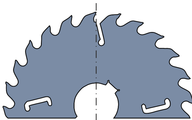
Joonis 1.39 Ketassae hammasvöö tsoonis paiknevatesse sisselõigetesse – termokompensaatoritesse – on kinnitatud külglõikurid. Külglõikurid on ka ketta tsentri pool asuvates jahutusavad. Joonis: juliautensili.com
