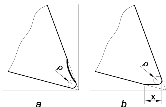
Joonis 1.31 Teriku geomeetria muutus: a – täispuidu lõikamisel, b – puitmaterjalide lõikamisel.
