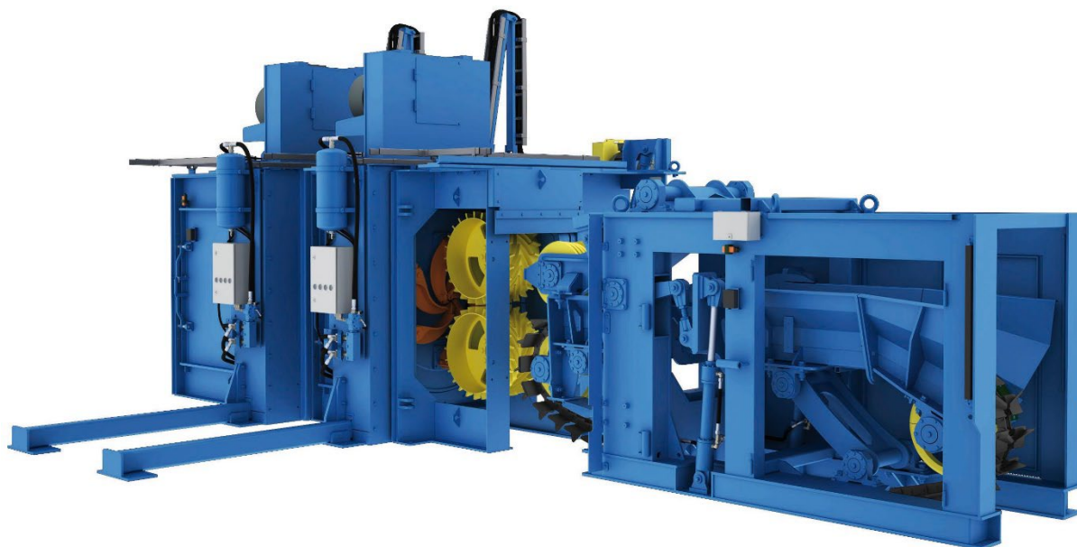
Joonis 2.12 Rootorkoorimispingi üldvaade (koorimispingi ees on renni ja nukkidega ketiga palgi tsentreerimisseade ja kollased etteandevaltsid) Foto: Valon Kone OY
