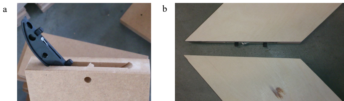
Joonis 9.27 Clamex 15 paigaldus tapipesasse: a – ja b – eeringliides. Fotod: K. Saar
