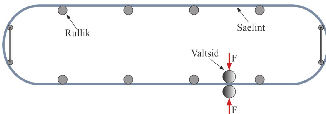
Joonis 1.45 Saelindi eelpingestamine valtsimise teel. Punased nooled näitavad valtside rakendatud survejõu suunda.
