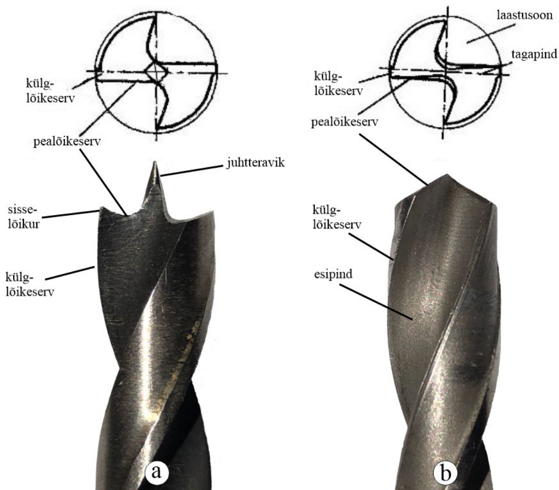
Joonis 1.80 Puidupuurid: rist- (a) ja pikikiudu (b) puurimise puuride elemendid.
