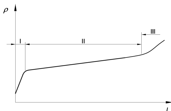
Joonis 1.32 Nürinemise etapid: I – sissetöötamine, II – monotoonne kulumine, III – katastroofiline kulumine.
