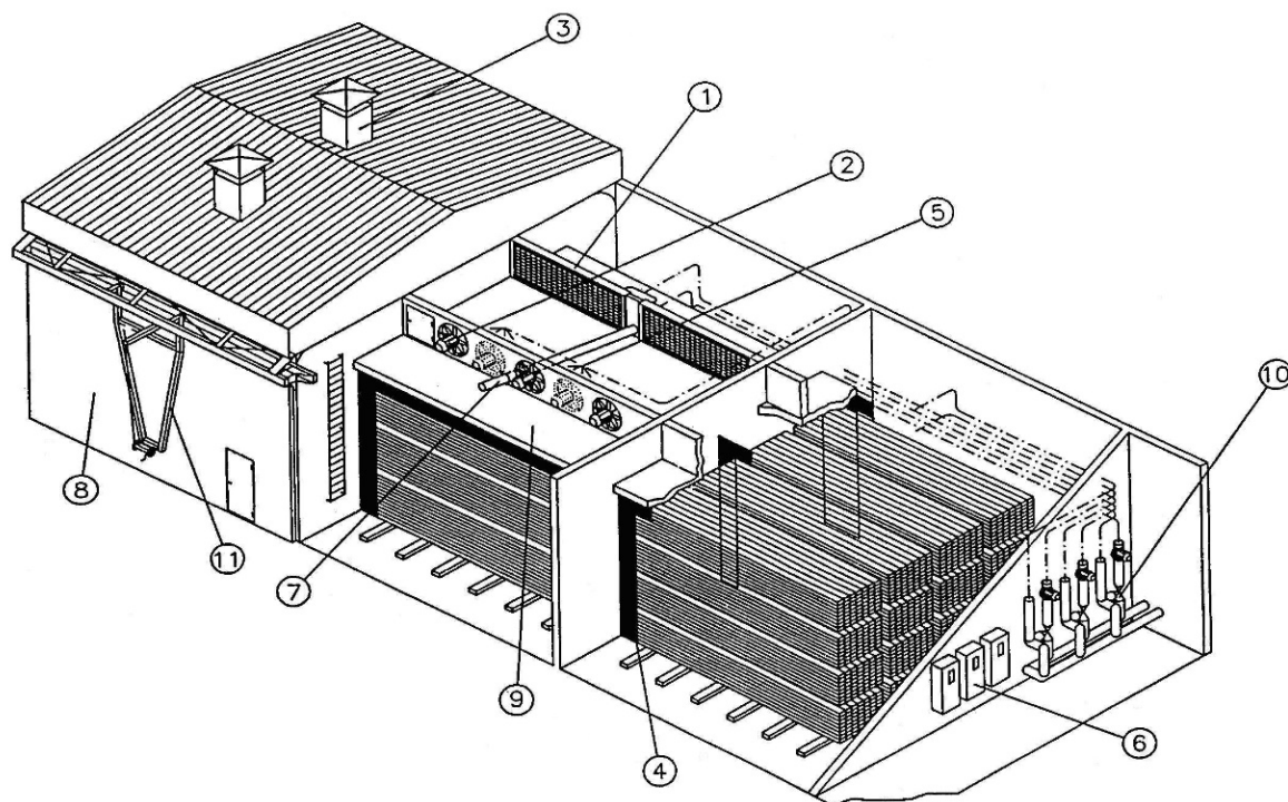
Joonis 3.5. AS Hekotek kamberkuivati: 1 – kalorifeer, 2 – ventilaator, 3 – õhuvahetuskanal, 4 – õhuvoolu tõkestusekraan, 5 – niisutussüsteem, 6 – juhtkilp, 7 – temperatuuri ja niiskuse andur, 8 – liuguks, 9 – vahelagi, 10 – ventiilid ja pumbad, 11 – ukse avamismehhanism.
