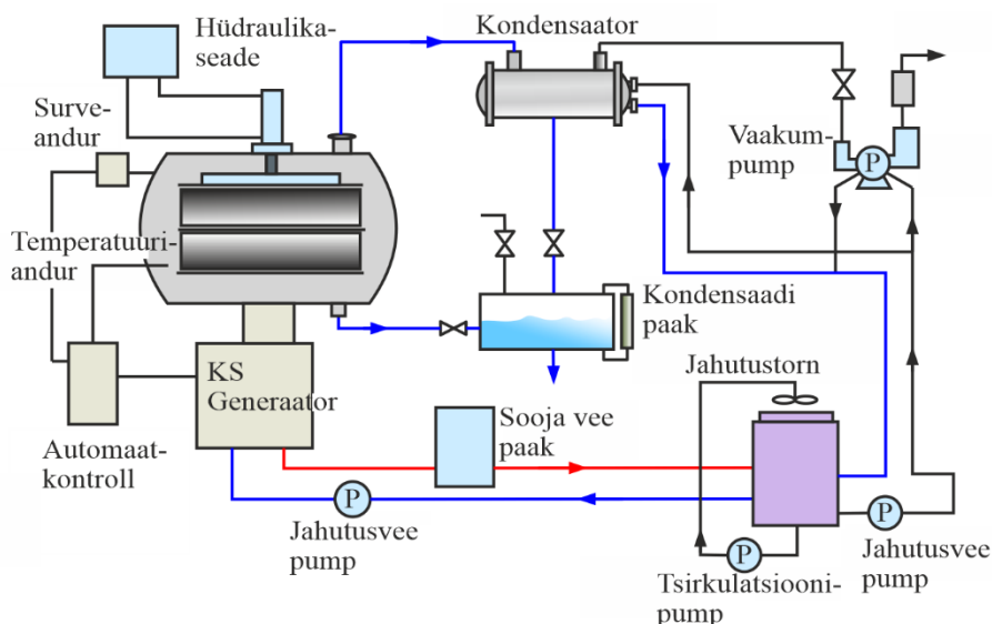
Joonis 3.28 Vaakumdielektrilise kuivatuse tehnoloogiline skeem.
