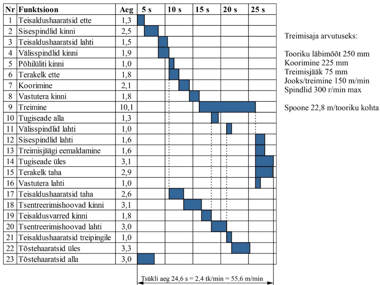
Joonis 2.72 Treimise etapid ja tööaeg.
