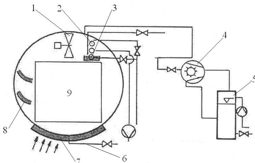
Joonis 3.26 Konvektiivse soojusülekandega vaakumkuivatuse skeem: 1 – ventilaator, 2 – kaloreifer, 3 – niisutusseade (aurusti), 4 – vaakumpump, 5 – veepaak, 6 – kondensaadi eraldus, 7 – jahutusõhu kanal, 8 – reguleeritav ekraan, 9 – materjalivirn.
