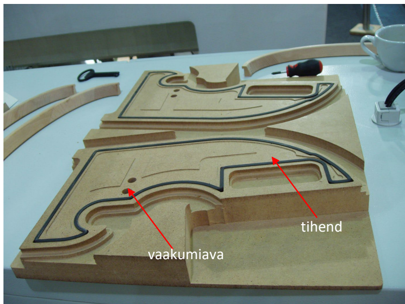
Joonis 4.9 Tooriku baseerimise ja kinnitusrakis CNC-töötluceskuses. Foto: Ü. Luga
