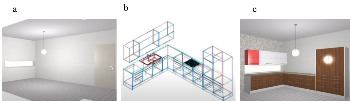
Joonis 10.5 IMOS 3D programmis loodud kööginõu: a) IMOS Plan ruumimudel, b) Article Designer sõrestikesitlusena kuvatav 3D-mudel ja c) IMOS Plan 3D-mudel.
