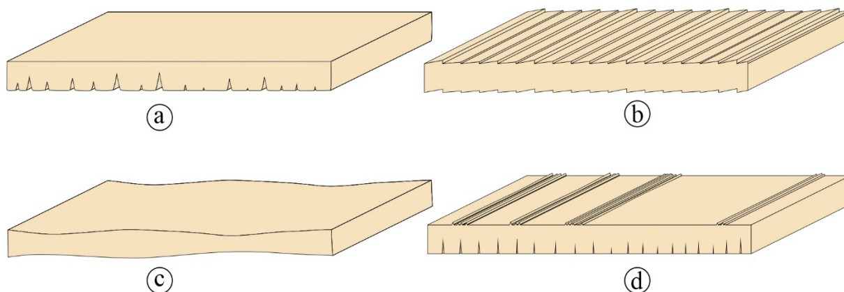
Joonis 2.85 Spooni defektid: a – spooni lõhenenud tagakülg, b – laineline spoon, c – lainelise spooni paksuse kõikumine, d – kare spoonipind.
