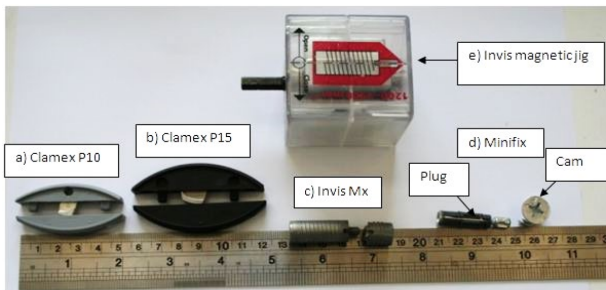
Joonis 9.34 Lahtivõetavate nurkliidete ja T-liidete koostamiseks kasutatavad liited: Clamex P10 ja P15 plastlamelltüüblid, Invis Mx kruvitüübel ja magnet tõmmits ning Minifix eksstsentrik-tõmmits.
