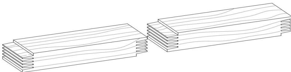
Joonis 4.18 Horisontaalsõrmtapp.
