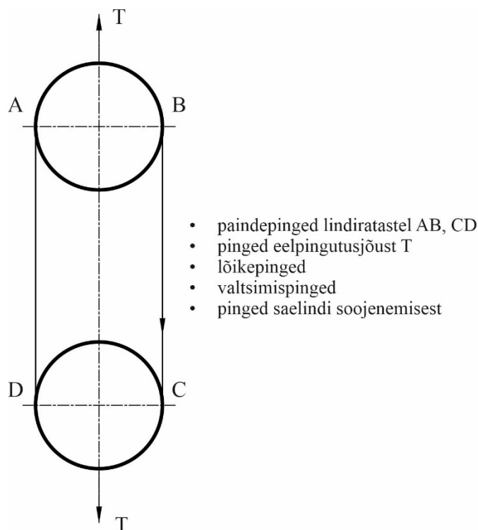
Joonis 1.44 Pinged saelindis.
