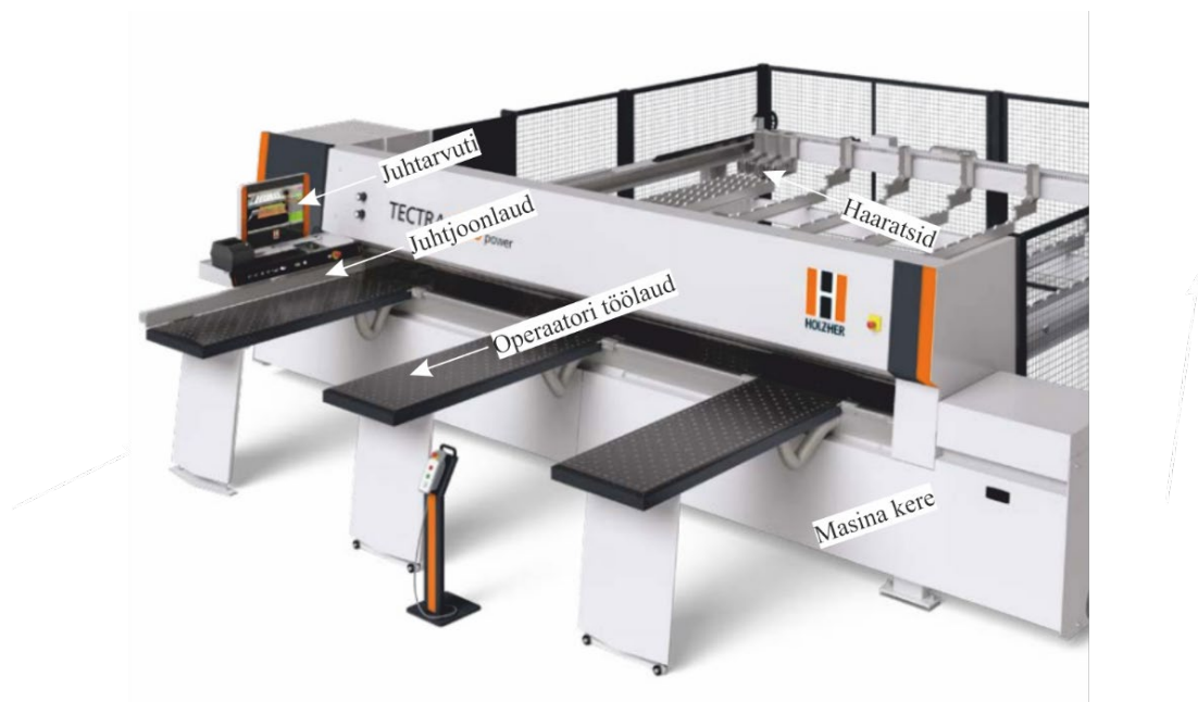
Joonis 6.3 Formaatsaag. Foto: HOLZ-HER GmbH
