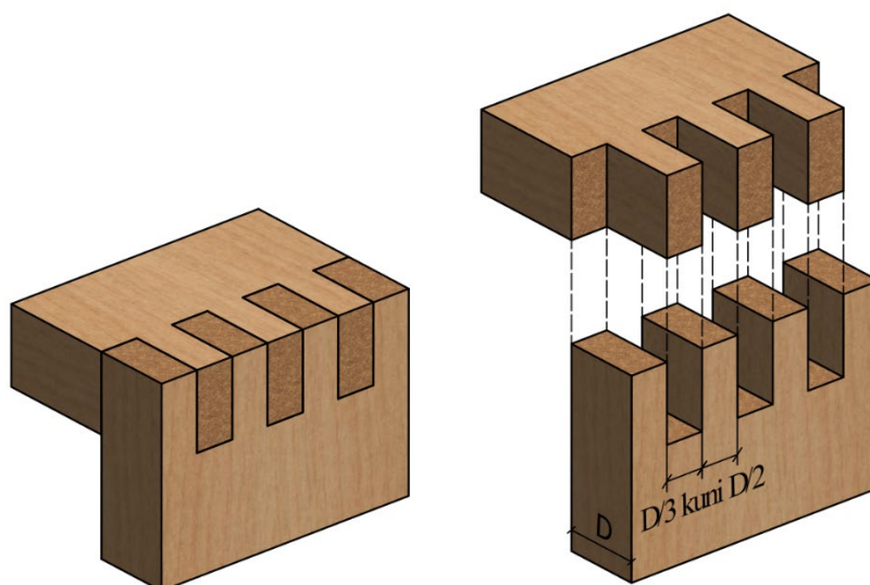
Joonis 9.44 Rööptapp.
