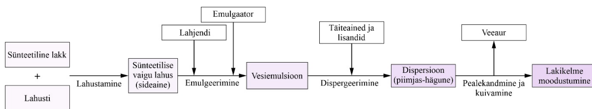
Joonis 8.30 Lakikile moodustumine vesialusel lakikihi kuivamisel.
