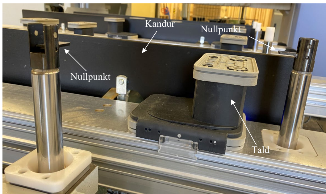
Joonis 7.40 Tekstoliidist kandurid, vaakumtallad, külgmised ja eesmised nullpunktid.
