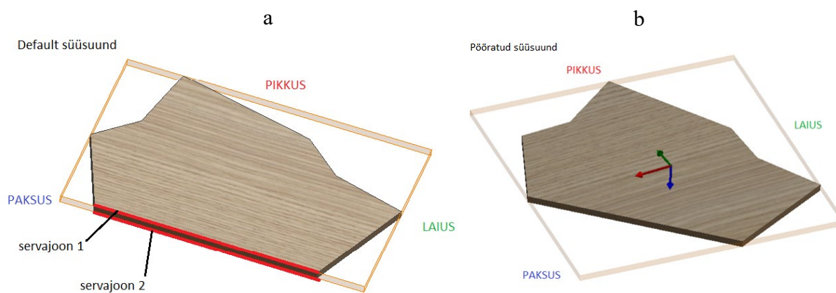
Joonis 10.18 Mööblidetaili pealistusmaterjali puidusüüsuund: a – vaikumisi ( default ) pikisüunas ja b – pööratud süüsuund. Autor: L. Link
