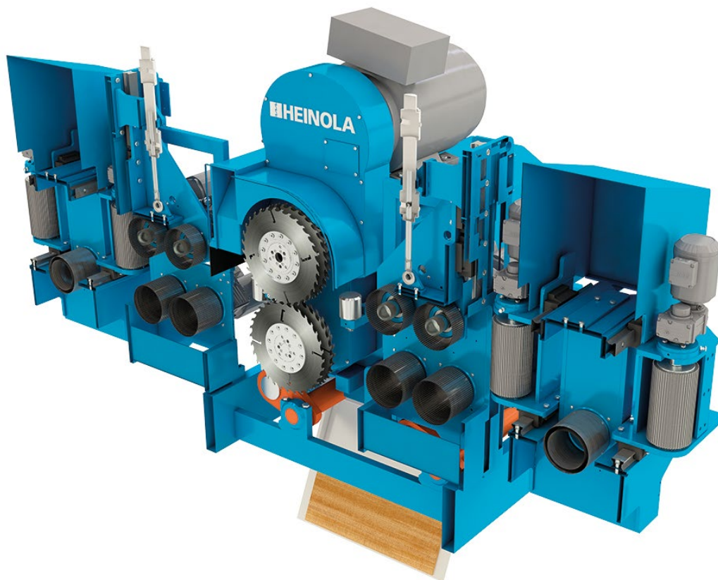
Joonis 2.43 Kahe sünkroonselt pöörleva saevõlliga prussisaag. Foto: Heinolan Sahakoneet OY
