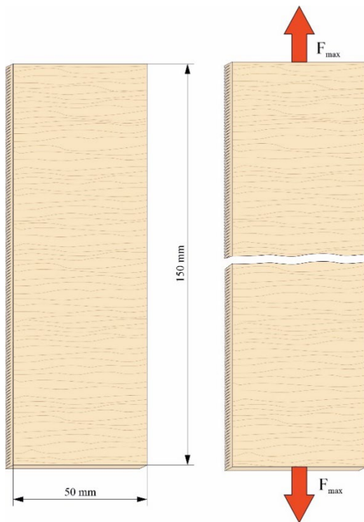
Joonis 2.87 Katsekeha spooni risttõmbetugevuse määramiseks.
