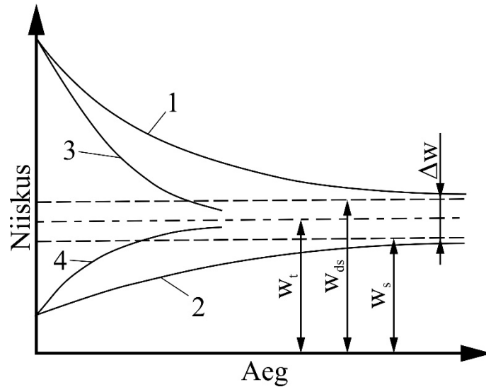
Joonis 3.1. Niiskuse sorptsiooni- ja desorptsioonikõverad: 1, 2 – vastavalt niiskuse desorptsiooni- ja sorptsioonikõverad saematerjalis, 3, 4 – vastavalt niiskuse desorptsiooni- ja sorptsioonikõverad peenestatud puidus.
