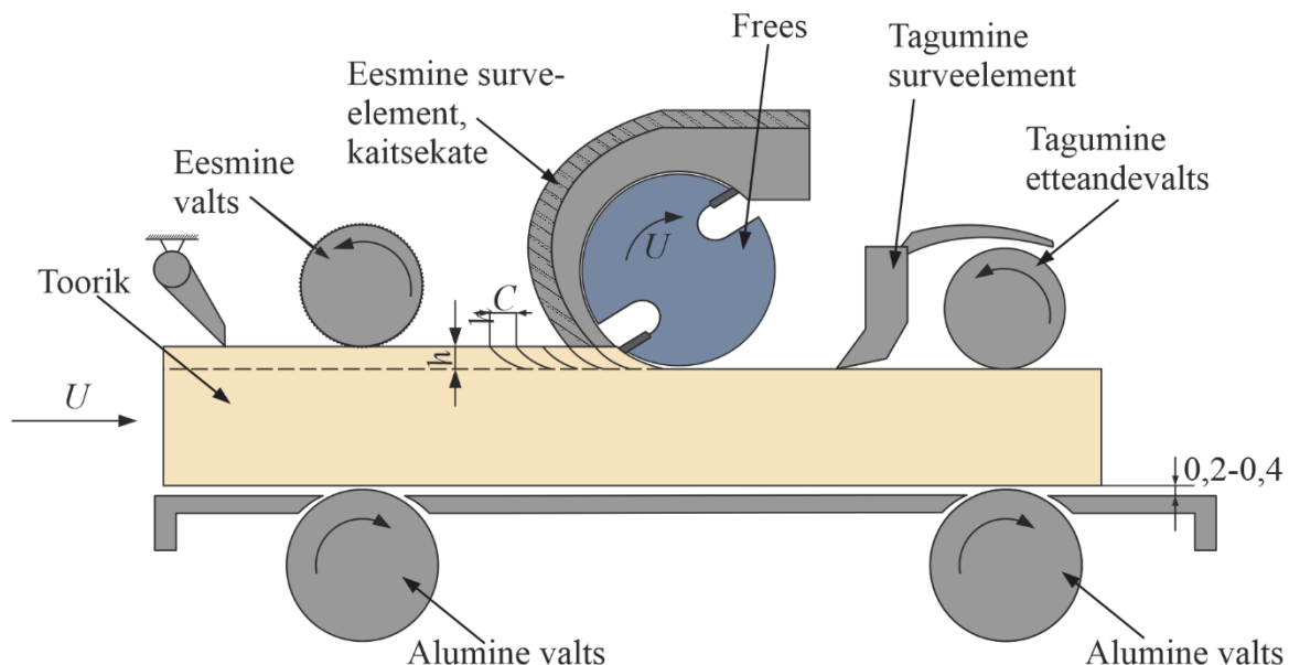
Joonis 1.74 Paksusmasina tööpõhimõte.
