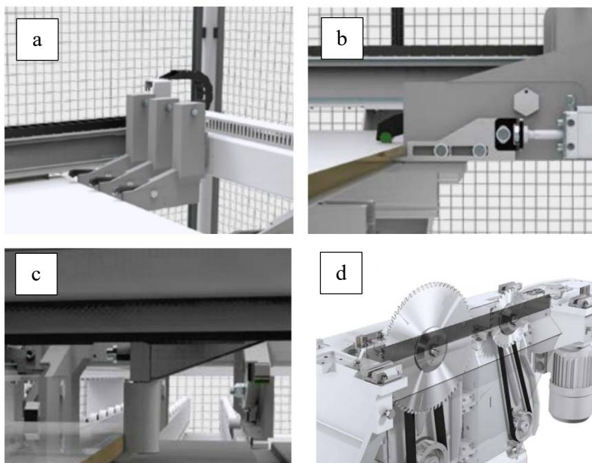
Joonis 6.4 Formaatsae agregaadid: a – haaratsid, b – haarats koos ülekatte detailide piirajaga, c – külmine surverull, d – saagimisüksus põhiketta ja ettelõikesaekettaga. Foto: HOLZ-HER GmbH
