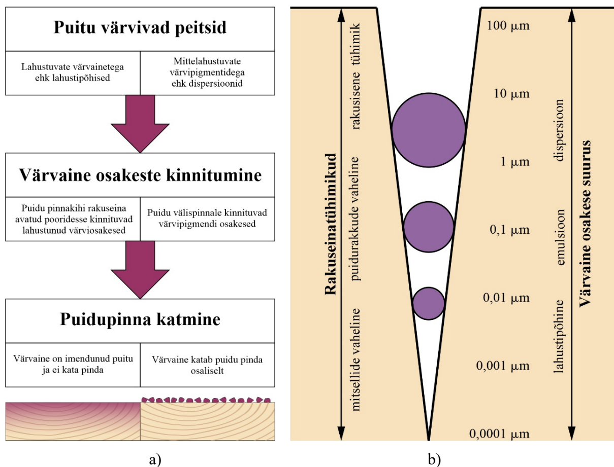
Joonis 8.10 Puituvärvivad peitsid ja värvaineosakeste suuruse võrdlus puidurakuseina tühimike suurusega: a – lahustipõhise ja dispersioonpeitsi võrdlus, b – puidurakuseina tühimike suurus võrrelduna peitsides/lakkides värviosakeste suurusega.
