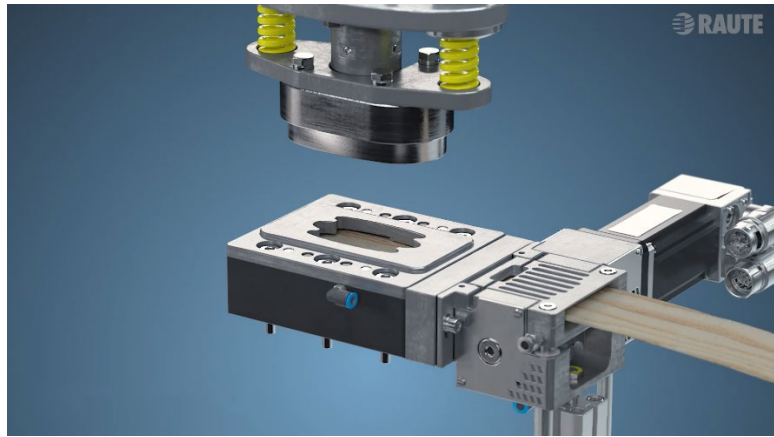
Joonis 5.58 Spooni paikamisseade. Allikas: Raute Oyj
