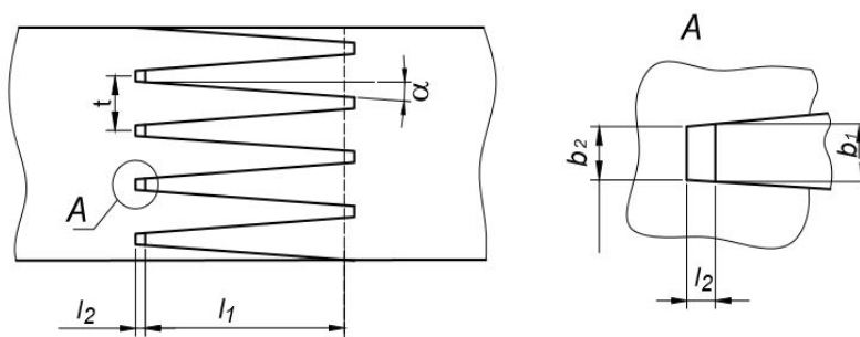
Joonis 4.17 Sõrmtappliite põhimõõtmed.
