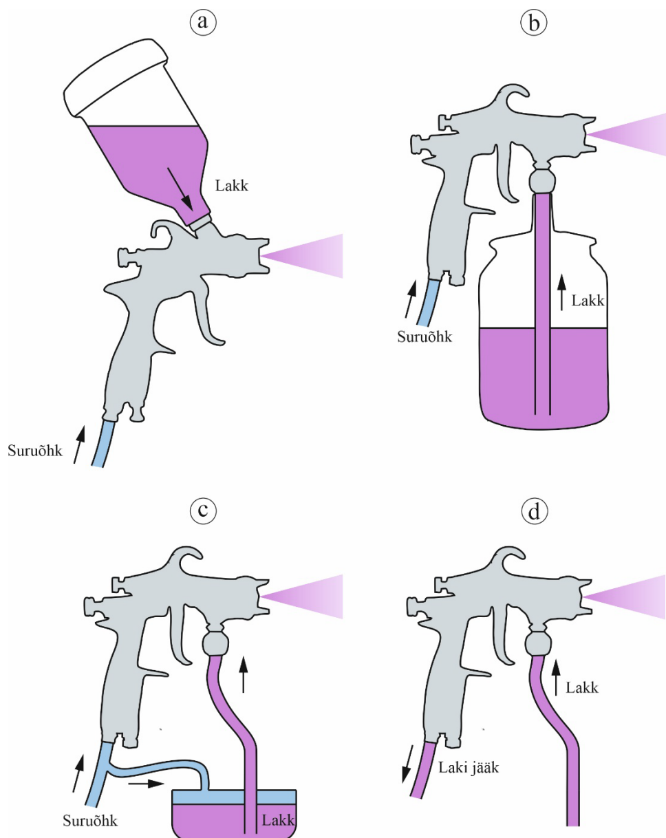
Joonis 8.44 Käsipihustusel kasutatavad laki etteandesüsteemid: a – ülaanumaga gravitatsiooni- line laki pealeandepüstol, b – alaanumaga ja laki alarõhuga kaasa imemisega püstol, c – surve- anumaga pealeandepüstol, d – pihustus laki pealeandega tsentraallakimahutist.
