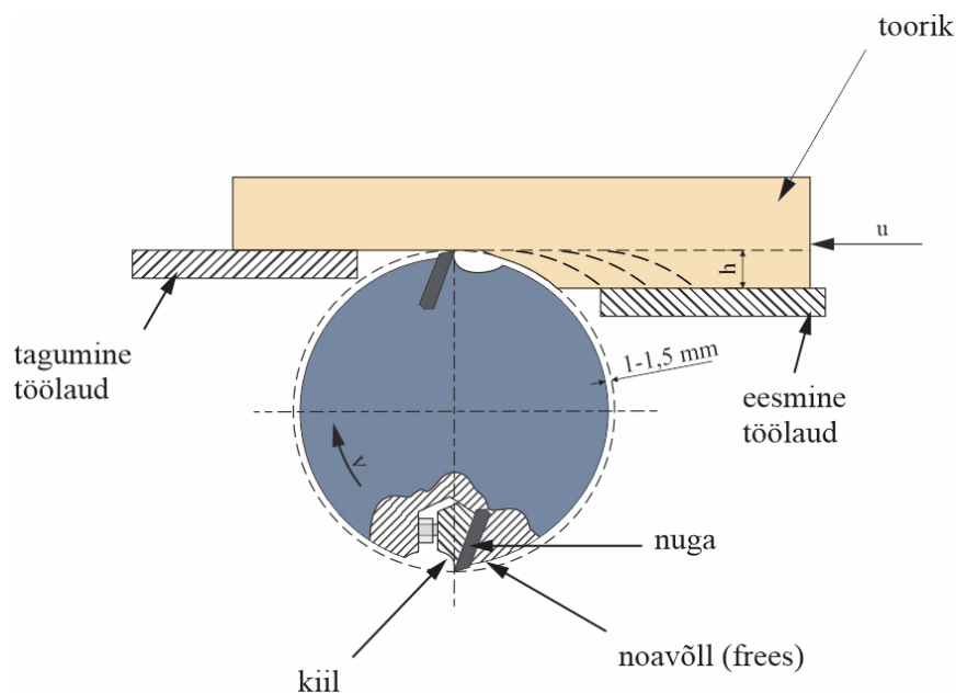
Joonis 1.73 Rihthõõvli tööpõhimõte.
