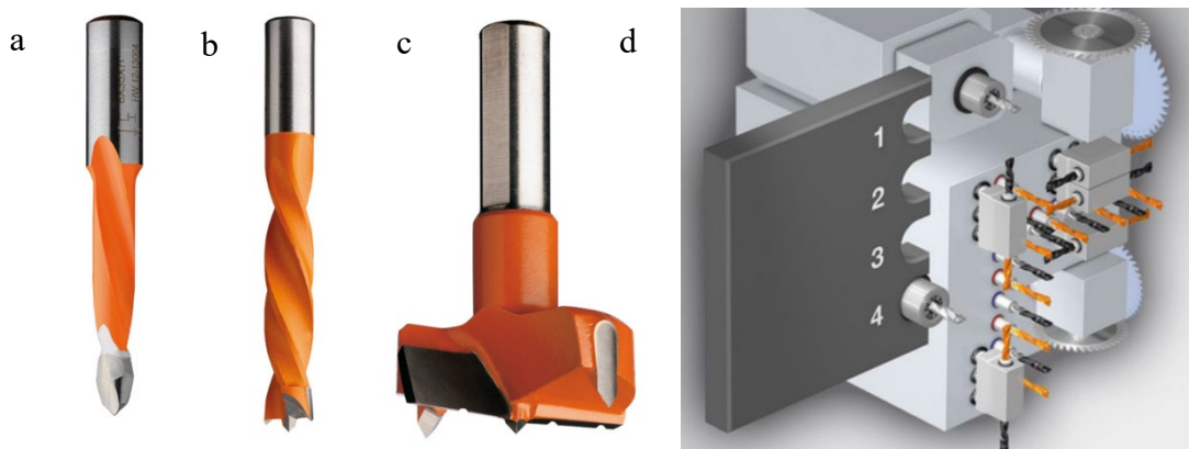
Joonis 7.25 CNC-pingi puurid: a – läbistav puur, b – mitteläbistav puur, c – mööblihinge pesa puur, d – vertikaalse CNC-masina tööriistad (oranžid puurid pöörlevad ühtepidi ja mustad vastupididi). Fotod: C.M.T. UTENSILI S.P.A & HOMAG Group AG
