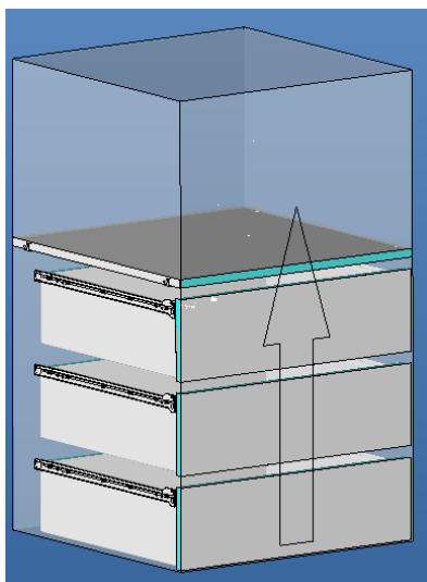
Joonis 10.38 Metabox-siinidega sahtlite komplekt. Rohelisega näidatud element on servakant. Autor: M. Muru
