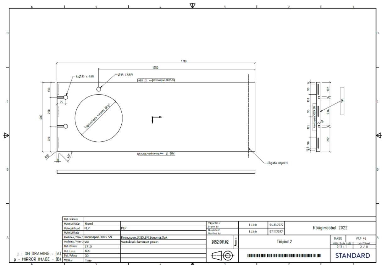
Joonis 10.24 Tööpinna detailjoonis. Autor: L. Link
