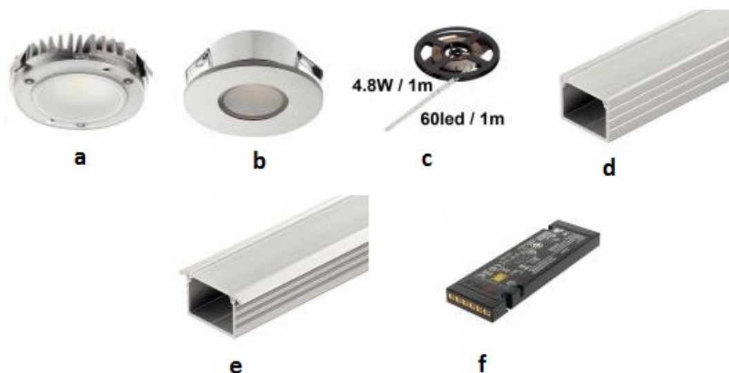
Joonis 9.75 Valgustid: a – pinnapealne kohtvalgusti, b – süvistatav kohtvalgusti, c – LED valgusriba, d – pinnapealne klaasiga profiil, e – süvistatav klaasiga profiil, f – transformaator.
