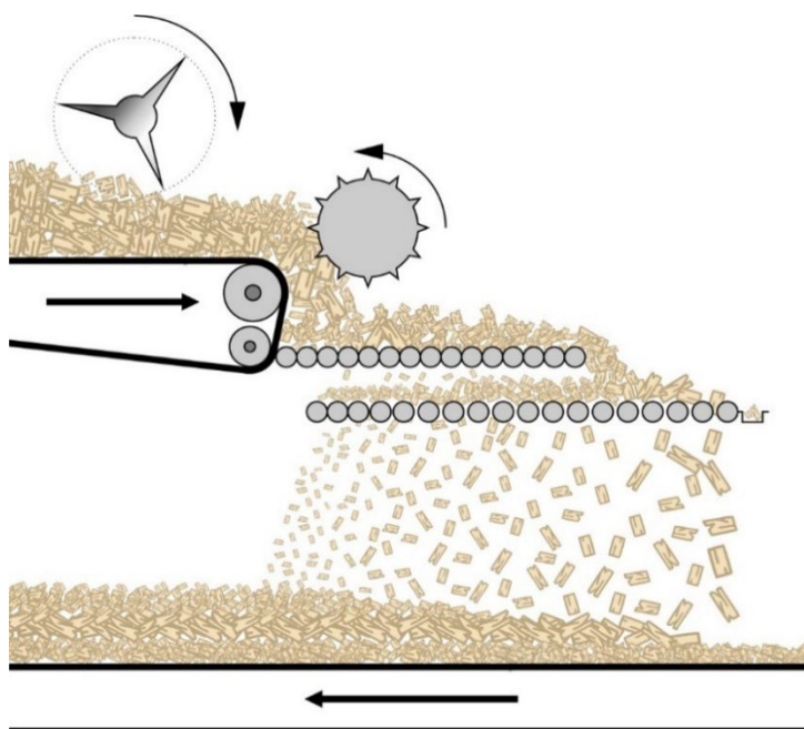
Joonis 5.86 Laastuvaiba moodustamine mehaanilise fraktsioneerimisega.
