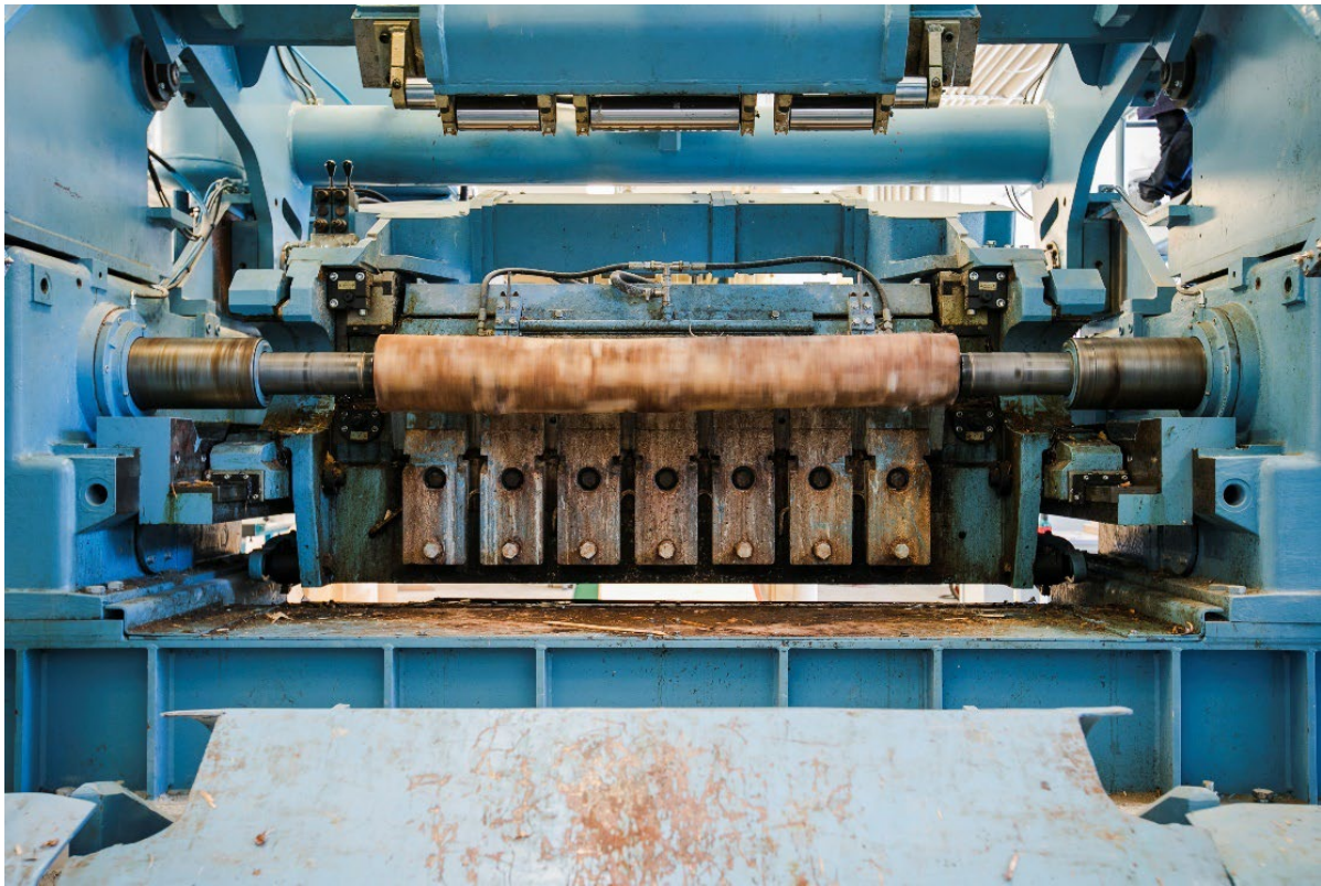
Joonis 2.66 Vineeritööstuses kasutatav spoonitreipink: pakk pöörleb spindlite vahel.
