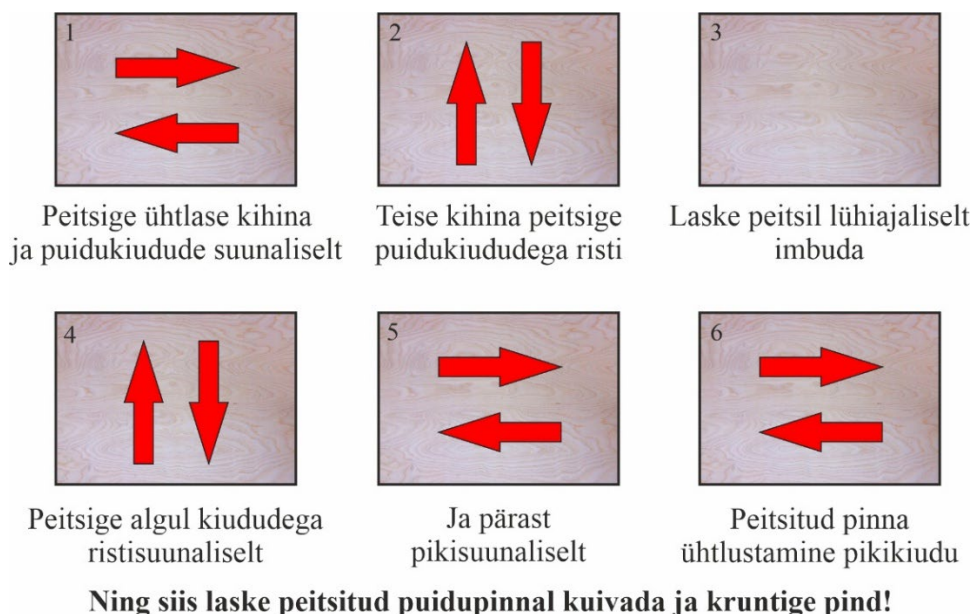
Joonis 8.12. Tööjärjekord puidupinna käsipeitsimisel.
