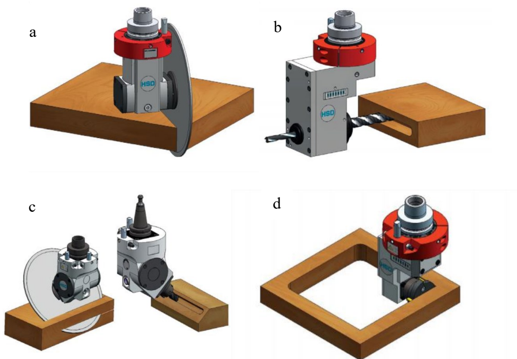
Joonis 7.20 Valik lisaagregaat: a – ristagregaat saega, b – ristagregaat puurimiseks ja freesimiseks, c – fikseeritud 45° nurgaga sae- ja freesagregaat ja d – nurgapuhastusagregaat. Fotod: HSD SpA
