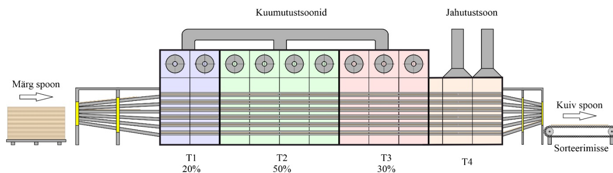
Joonis 3.36 Rullkuivatuslini tsoonid.
