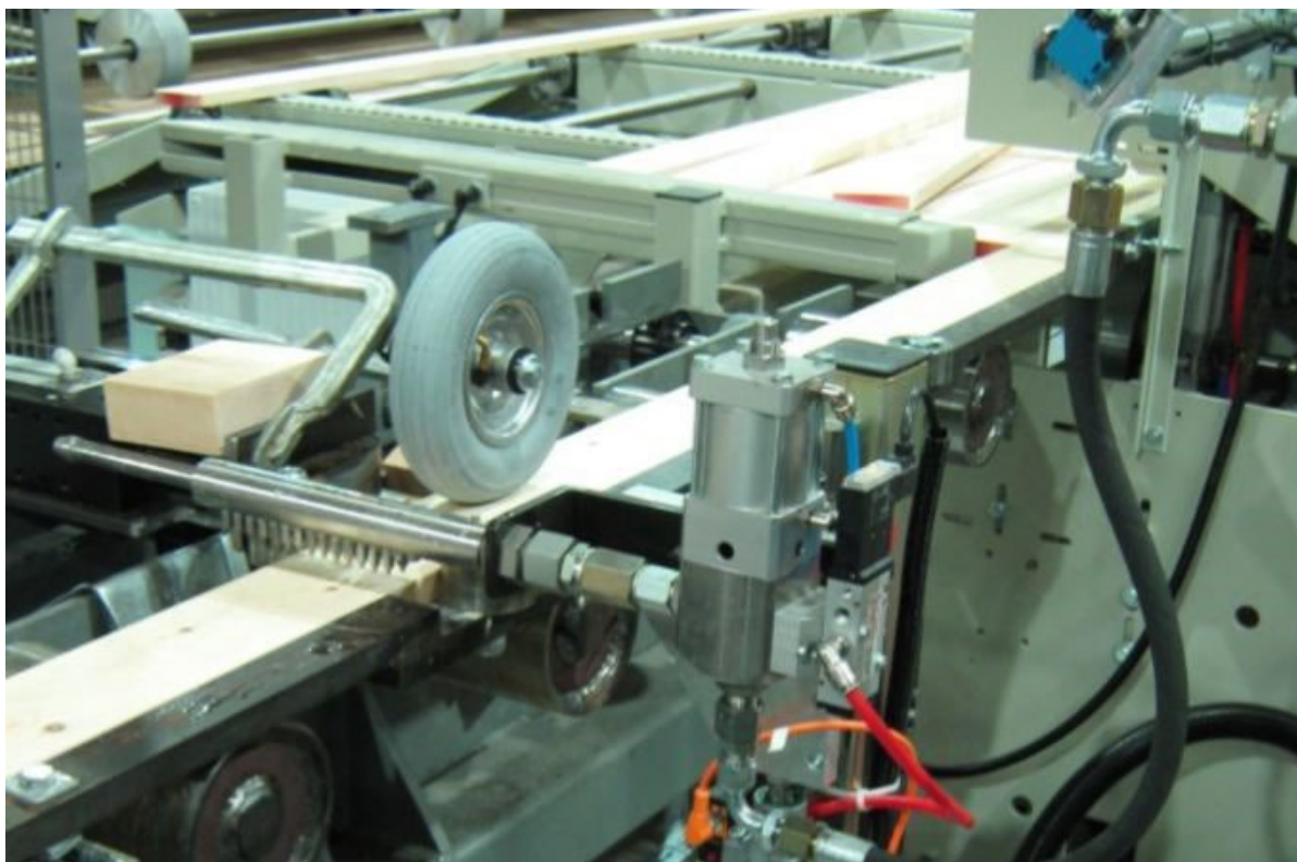
Joonis 5.9. Start-stopp-süsteemiga kardin-tüüpi liimitamisseade Foto: Mixon AB
