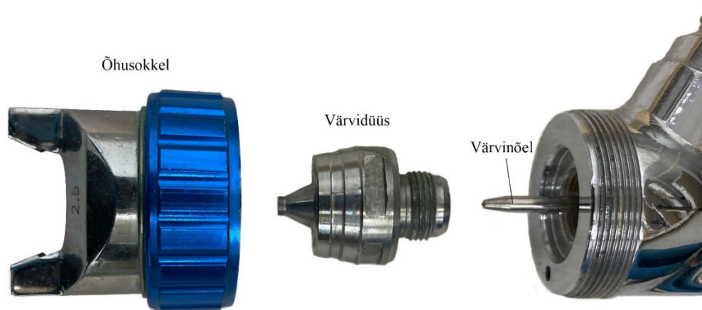
Joonis 8.48 Käsipihustuspüstoli õhusokkel, värvidüüs ja värvinõel.
