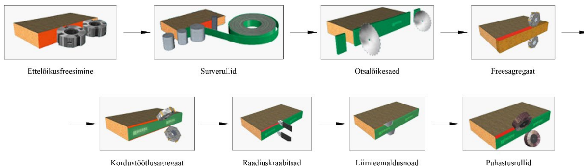
Joonis 6.22 Võimalik servapealistusmasina konfiguratsioon Foto: BIESSE S.P.A.
