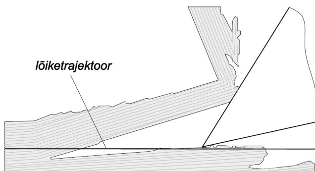
Joonis 1.24 Laastu moodustumine pikilõikamisel.
