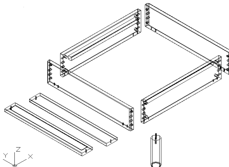
Joonis 10.1 AutoCAD-i sõrestikesitlusena kuvatud tumbadetailid. Autor: S.Vahemäe
