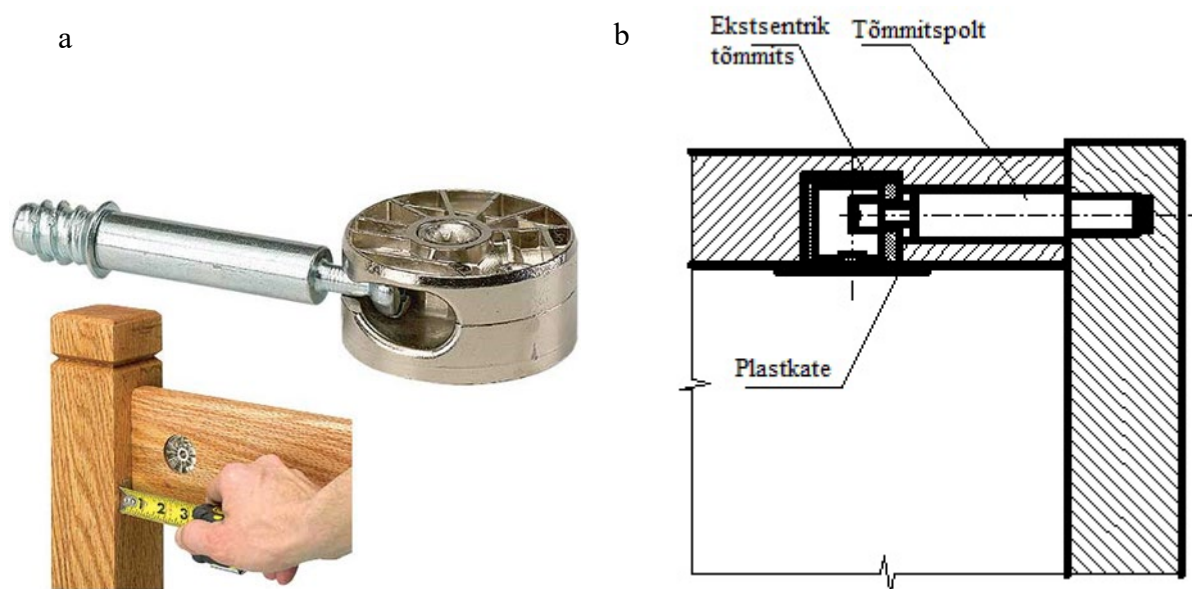
Joonis 9.16 Ekstsentriskõmmitsaga lahtivõetav liide: a – ekstsentriskõmmits ja koostatud liide, b – laeliide lõikes.
