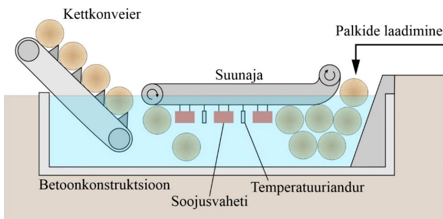
Joonis 2.58 Vee alla surutud palkidega bassein.
