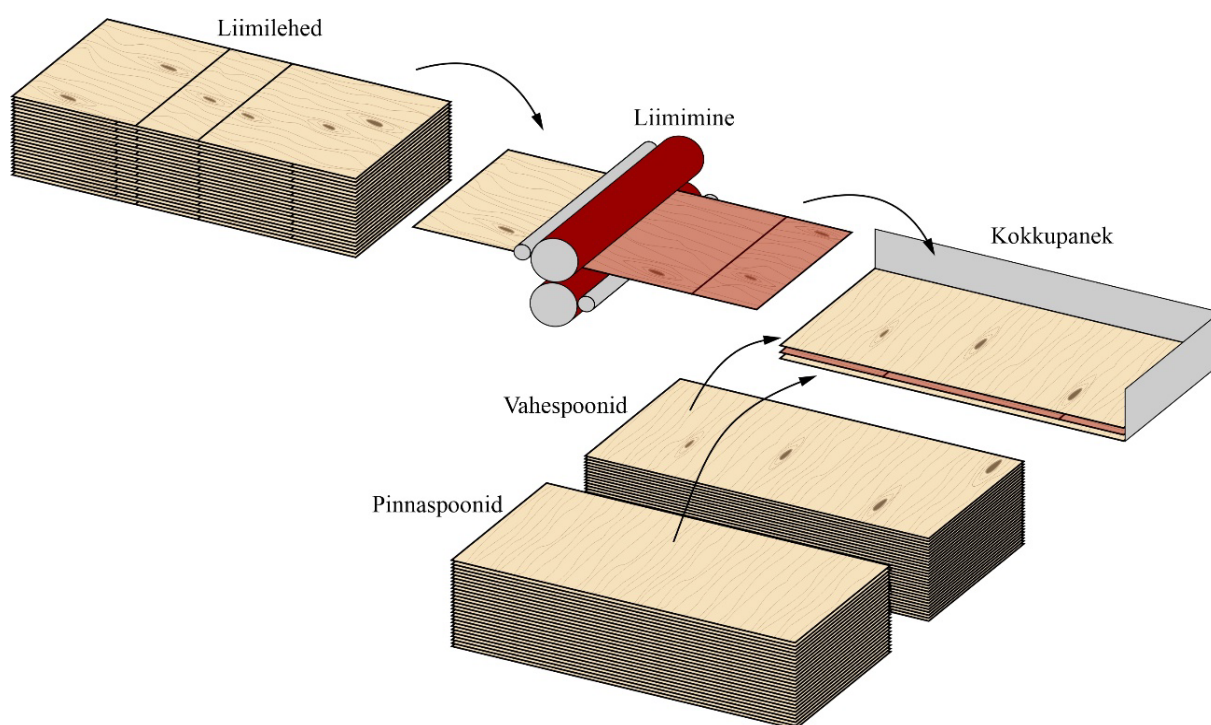
Joonis 5.71 Vineeritoorikute koosteskeem.
