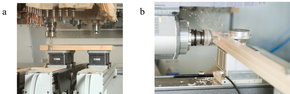
Joonis 7.5 Vaakumkonsoolile kinnitatud vaakumpadi (a) ja vaakumklamber (b). Fotod: J. Schmalz GmbH
