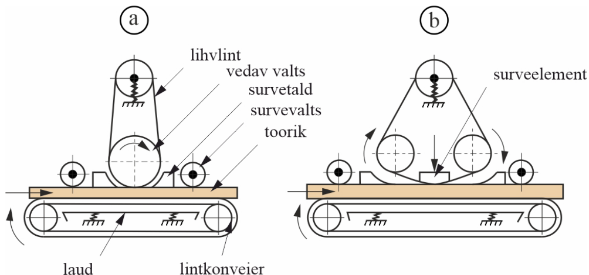
Joonis 1.98 Lailintlhvagregaadid: a – kontaktvaltsiga, b – surveelemendiga.
