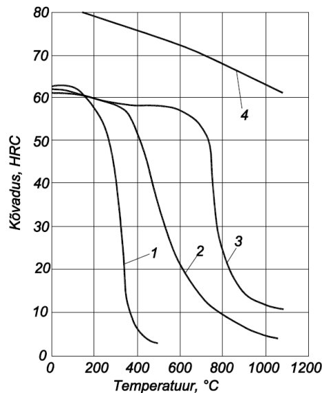
Joonis 1.28 Materjalide kõvadus: 1 – süsiniktööriistateras, 2 – poolsoojuskindel legeerteras, 3 – kiirlõiketeras, 4 – kõvasulam WC baasil.
