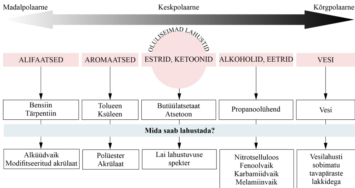
Joonis 8.21 Lahustite polaarsus ja kilemoodustajate (sideainete) lahustuvus.
