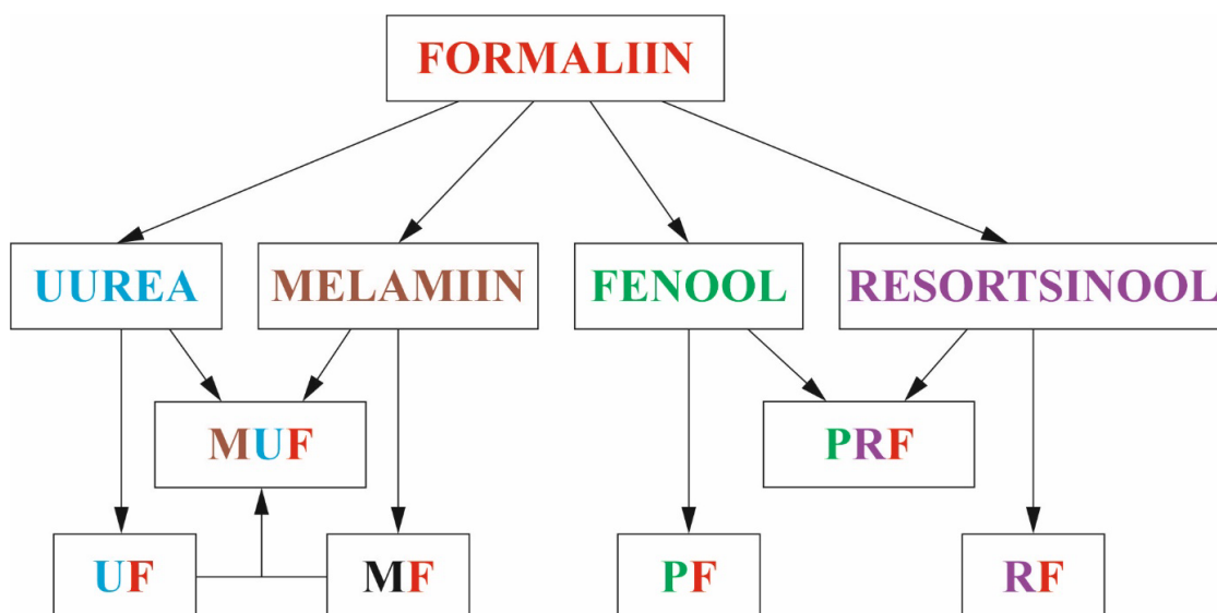
Joonis 5.6 Formaldehüüdliimide liigitus.
