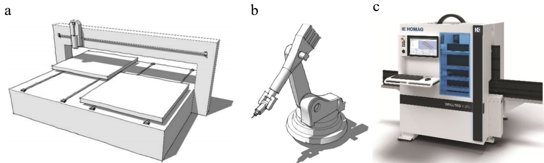
Joonis 7.4 Pendellauaga pink (a), kuueteljeline tööstusrobot (b) ja vertikaalne CNC-töötlemiskeskus (c). Joonis: A. Albert. Foto: HOMAG Group AG
