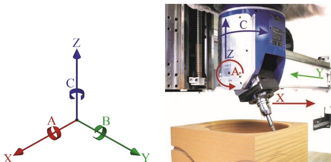
Joonis 7.2 CNC-töötlemiskeskuste vabadusastmed ja vabadusastmed viieteljelisel pingil. Joonis: K. Kiiman. Foto: HOMAG Group AG
