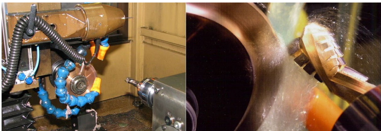
Joonis 1.34 Elektroerosioonterituspink. Fotod: M. Riistop ja J. Ingelman
