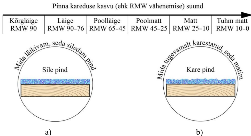
Joonis 8.37 Viimistletud puidupinna töötlemismeetodid: a – kõrgläike või b – tuhmi mattpinna saavutamiseks ja pinnakareduse RMV (reflektomeetri) mõõteväärtused kõrgläikest tuhmi matini.
