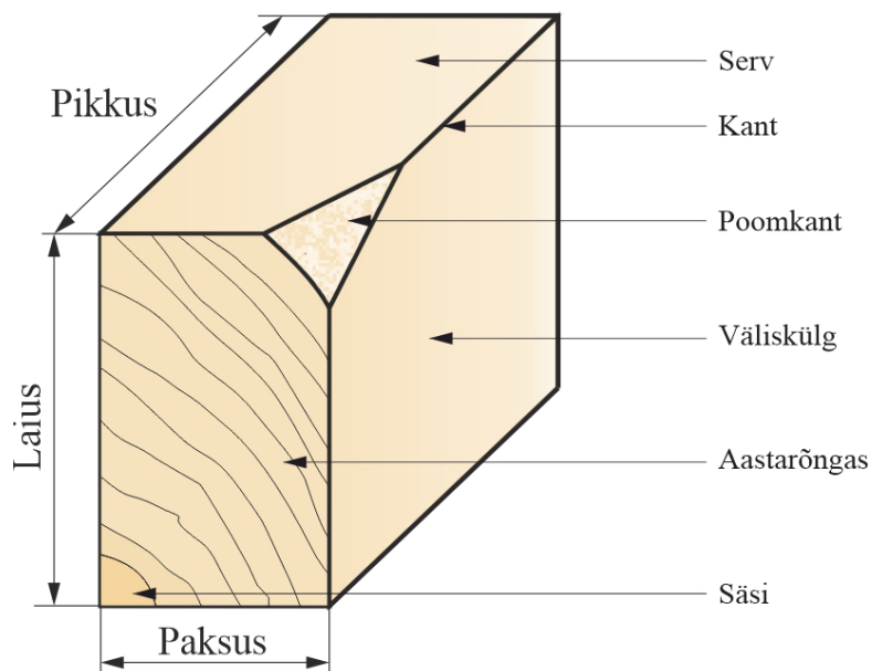
Joonis 2.28 Saematerjali geomeetrilised elemendid.
