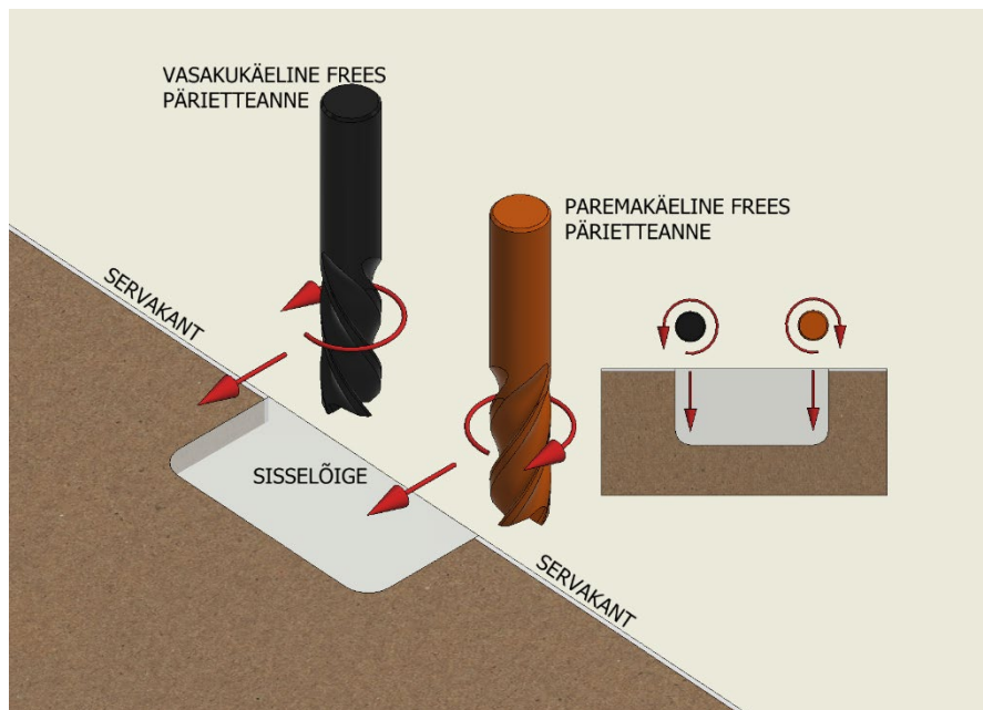
Joonis 7.19 Sisselõike tegemine kanditud servaga detaili. Joonis: K. Kiiman
