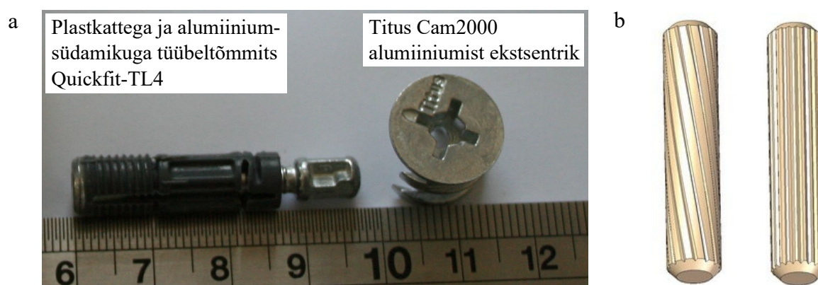
Joonis 9.18 Liitekinnitusdetailid: a – Titus Minifix tüübeltõmmits koos ekstsentriskuga, b – kõvast lehtpuidust (kask, pöök) kald- ja pikisoontega tüüblid.
