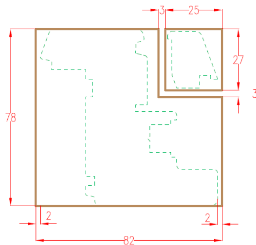
Joonis 7.55 Saksa-tüüpi puitakna tiivaprofiili toorik enne töötluskeskusesse minekut (töötlusvaru külgedelt 2 + 2 mm, klaasiliistu toorik 25 × 27 mm on eemaldatud eeltöötlemise käigus nelikanthöövelpingis).
