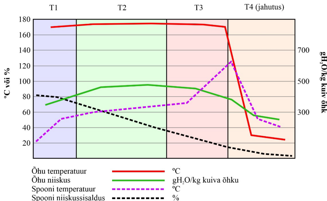
Joonis 3.44 Spooni kuivatusprotsessi neli etappi ehk tsooni.
