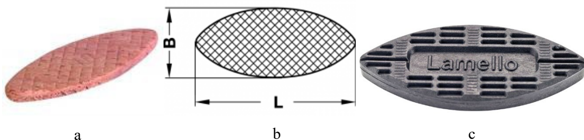
Joonis 9.39 Lamelltüüblid: a – puitlamelltüübel, b – lamelltüüblite mõõtmete tähistused, c – plastlamelltüübel paksusega 7 mm detailide joondamiseks ja ühendamiseks.
