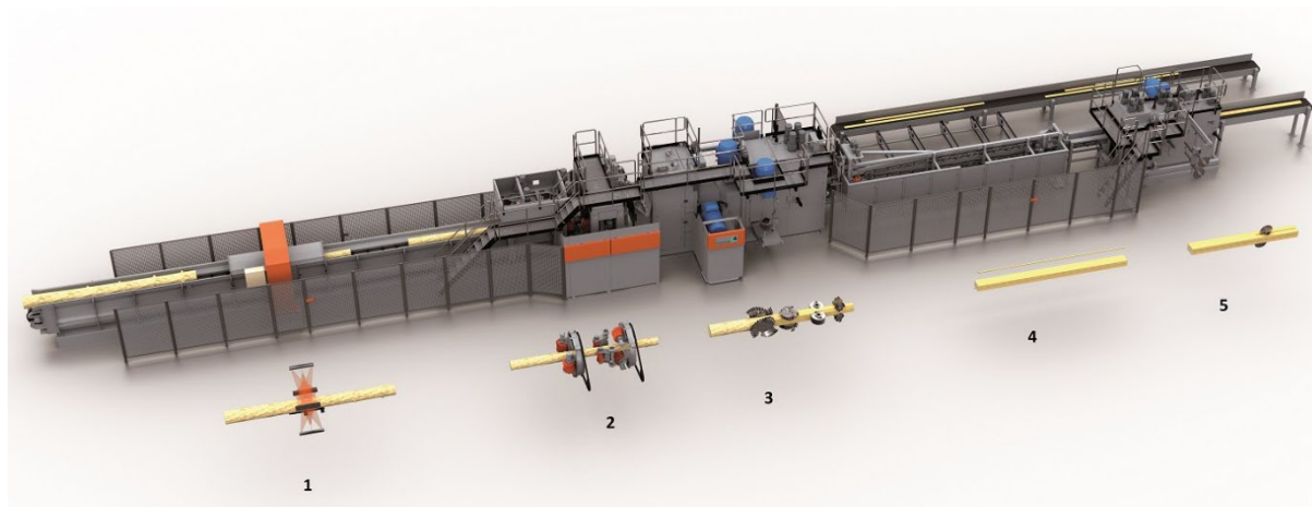
Joonis 2.39 Saeliin HewSaw R250A.1.2: 1 – palgiskanner, 2 – kahe rootoriga palgi pikitelje ümber pööramise seade (vt joonis 2.30); 3 – saagimisseade (vt joonis 2.38); 4 – seade küljelaudade eraldamiseks; 5 – prussisaag. Foto: Veisto OY
