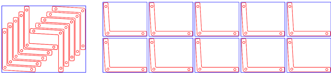
Joonis 7.7 L-kujuga detailide töötlemine nesting -meetodil ja nesting -meetodita. Joonis: K. Kiiman
