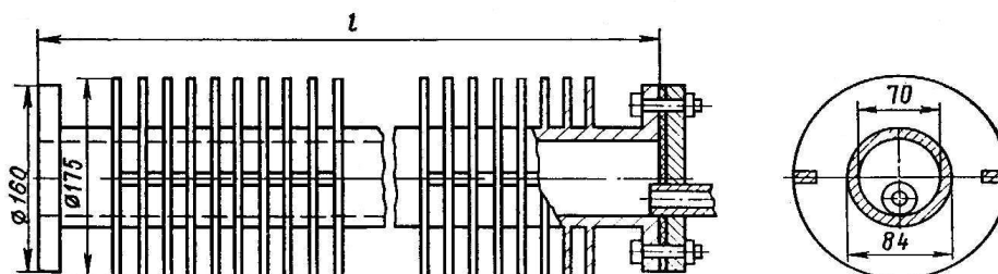
Joonis 3.10. Suuremõõtmeline kalorifeeri ribitoruelement.
