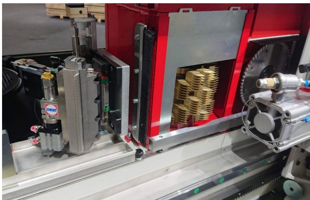
Joonis 4.22 Pakett-tüüpi sõrmjätikuseade ettelõikussaa (paremal), sõrmtapi freesid (keskel) ja metallist kamm liimi pealekandmiseks (vasakul). Foto J. Salla
