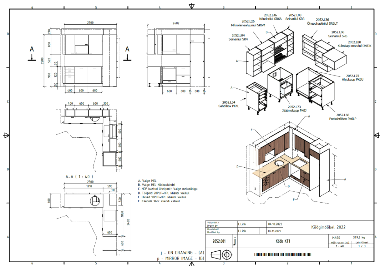
Joonis 10.23 Woodwork for Inventoris vormistatud köögi üldvaate joonis. Autor: L. Link
