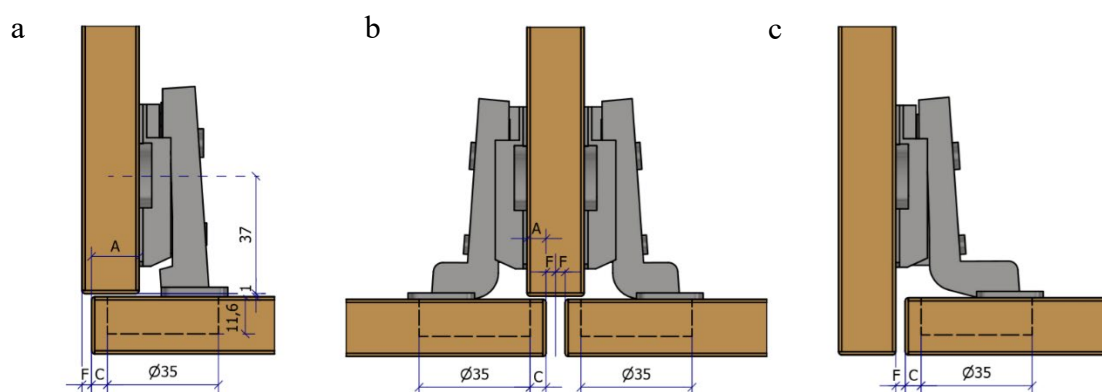
Joonis 9.50 Eri tüüpi uksehinged: a – pealekäiv hing, b – poolpealekäiv hing, c – sissekäiv hing (hingede avanemisnurk on \sim 110^\circ ). Joonis: M. Mäetalu
