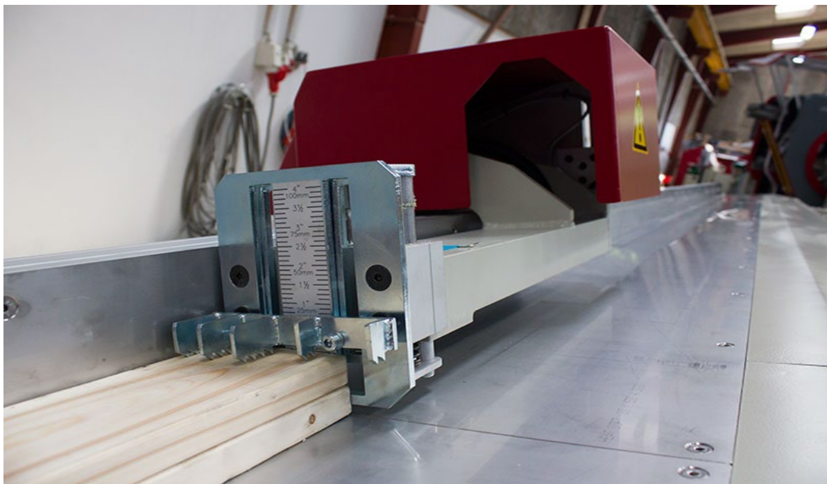
Joonis 4.27 Optimeeriva järkamissaet tõukur. Foto: System TM
