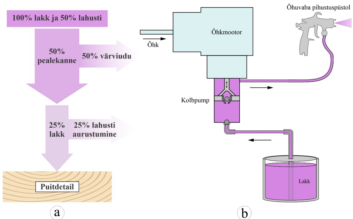
Joonis 8.47 Lahustipõhise laki käsipihustamine suruõhuga puitdetailile (a) ja laki pihustamine kõrgsurvega õhuvaba pihustussüsteemiga (b).
