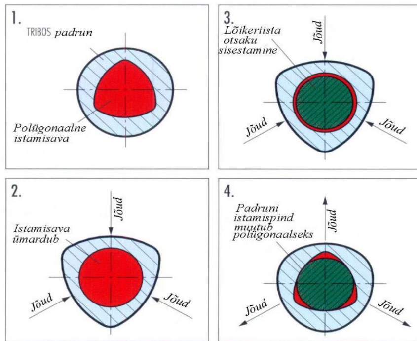
Joonis 1.68 Tribos-kinnituspadrundi tööpõhimõte.
