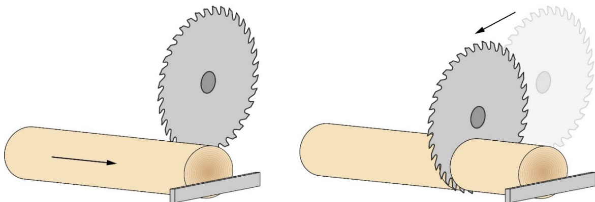
Joonis 2.61 Palkide spoonitoorikuteks järkamine pendelsaega.
