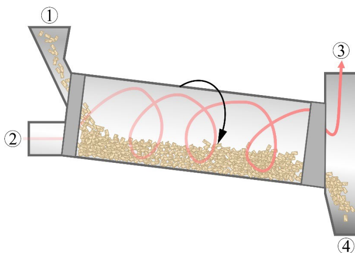
Joonis 3.48 Trummelkuivati: 1 – toitesead, 2 – küttekolle, 3 – gaasikäik kuivatusagensi retsikulationiks, 4 – kuivatatud laast välja.
