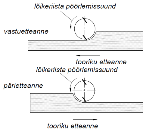
Joonis 1.9 Päri- ja vastuetteanne.
