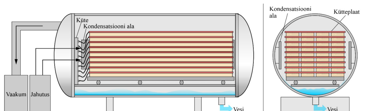
Joonis 3.27 Konduktiivse soojusülekandega vaakumkuivati.
