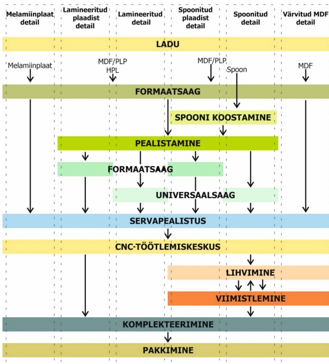
Joonis 6.1 Plaatdetailide töötlemise operatsioonid. Joonis: K. Kiiman
