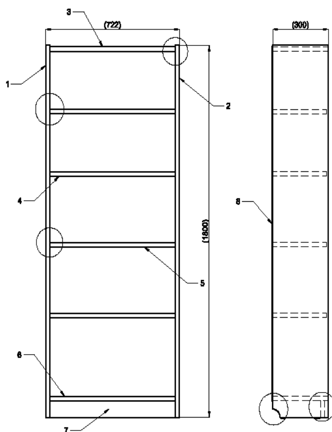
Joonis 9.80 Raamaturiiuli eest- ja külgsuuna gabariitmõõtmega.
