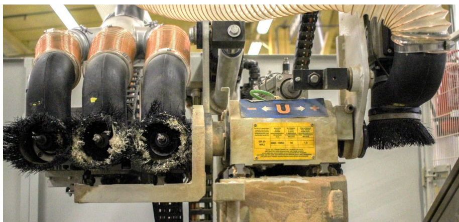
Joonis 7.46 Kahe suporti ja nelja mootoriga CNC-pink lengide töötlemiseks.
