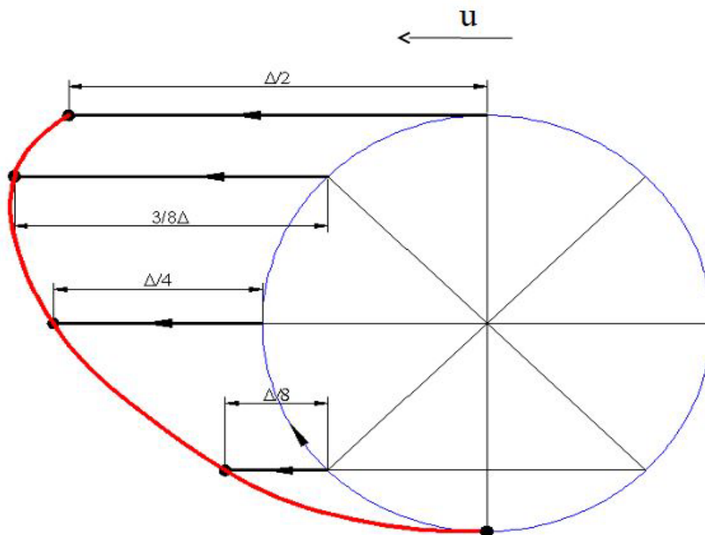
Joonis 1.52 Freesimise lõiketrajektoori kujunemine ühe lõiketeraga freesi korral.
