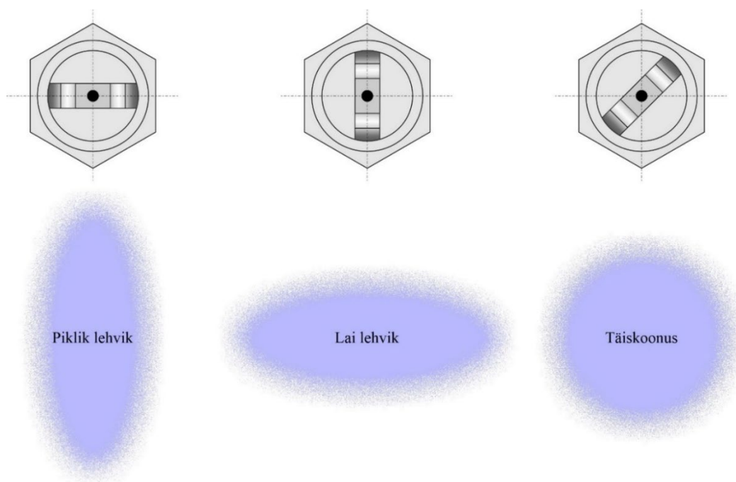
Joonis 8.49 Pihustuslehviku kuju reguleerimine käsipihustusel lakipüstolist.
