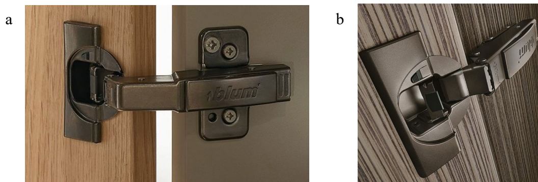
Joonis 9.49 Mööblihinge kinnitus: a – tasapindne T-tallaga hing ja b – pealekäiv sirgetallaga hing. Fotod: BLUM
