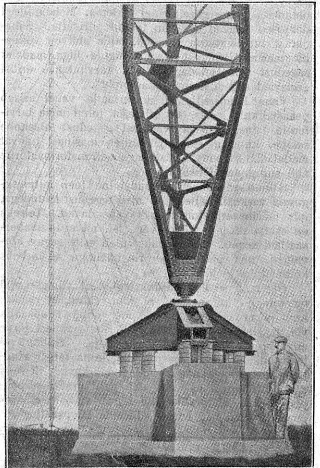
Coltano raadiojaama 220 m. kõrgused antennimastid.
