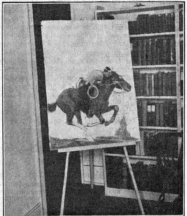
Ameeriklased on teinud huvitava kombinatsiooni valjuhääldajast ja õlimaalist. Huvitav on siinjuures see, et valjuhääldaja koonus on peidetud lasso-rõngasse.
