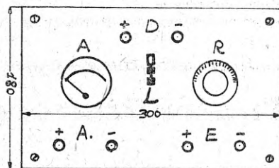
Lülitustahvel.
