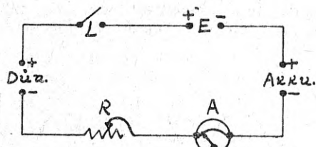
Lülitustahvi skeem.
