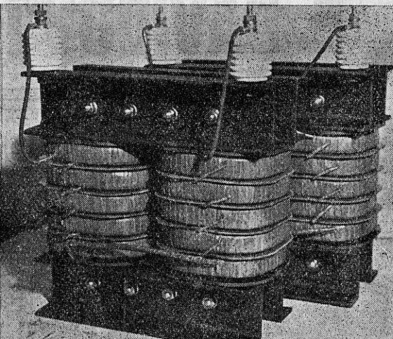
Modulatsiooni drossel Tallinna saatjale
