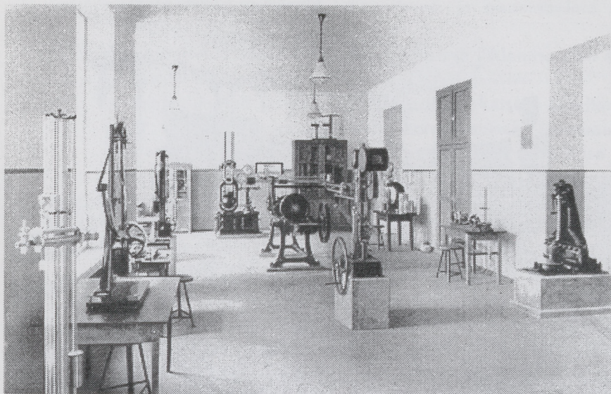
Tugevus- ja tehnilise mehaanika laboratooriumi väike masinaruum.
