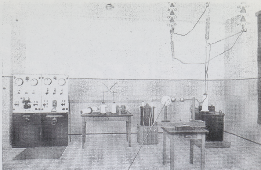
Elektrotehnika laboratooriumi kõrgepingeruim.
