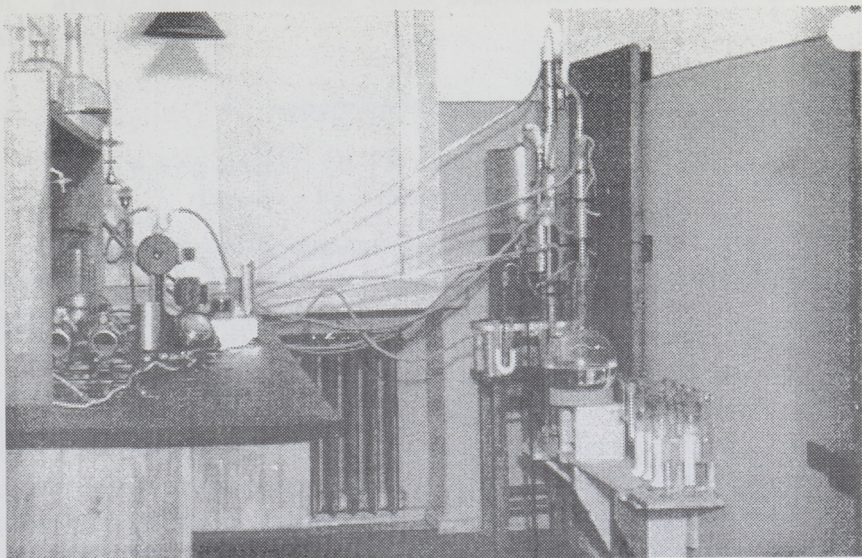
Füüsikalise keemia laboratooriumi juhtivusvee destillatsiooni seadeldis.
