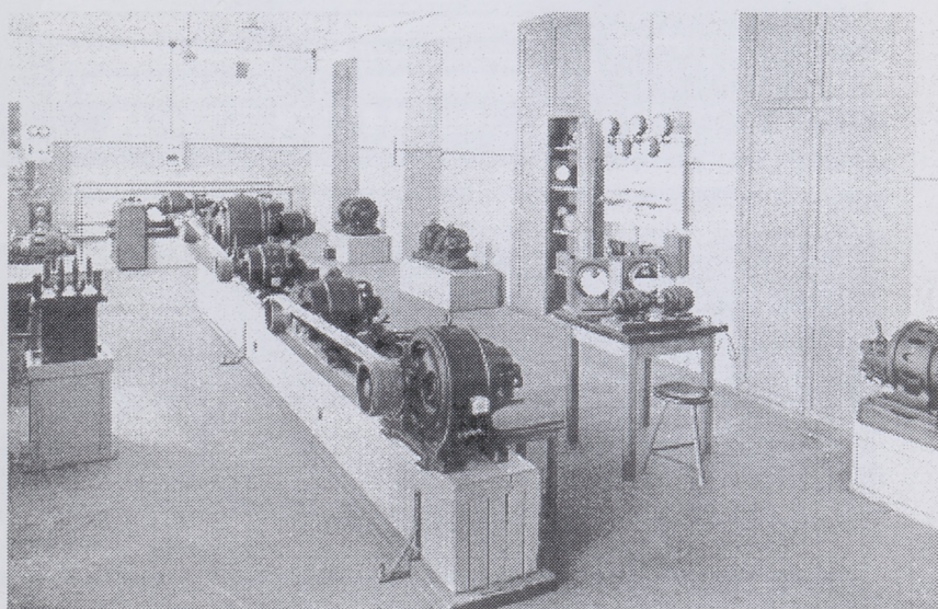
Elektrotehnika laboratooriumi masinaruum.
