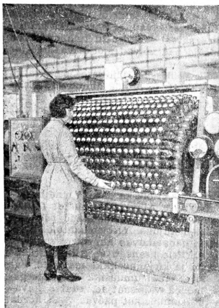
N. n. „põletisraam“, mille abil kuumutatakse lampe enne proovimist
