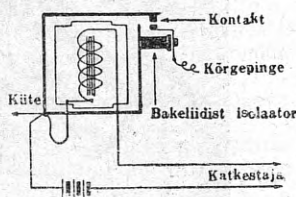
Joonis 5. Katkestaja relee, mis pannakse tegevusse käsi-katkestajaga madalpinge ahelas
