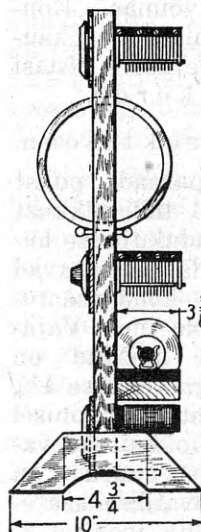
Joonis 2. Saateaparaat külje pealt vaadatuna
