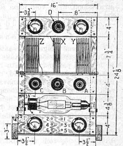
Joonis 3. Saateaparaadi konstruktsioon ja osade asetatus
