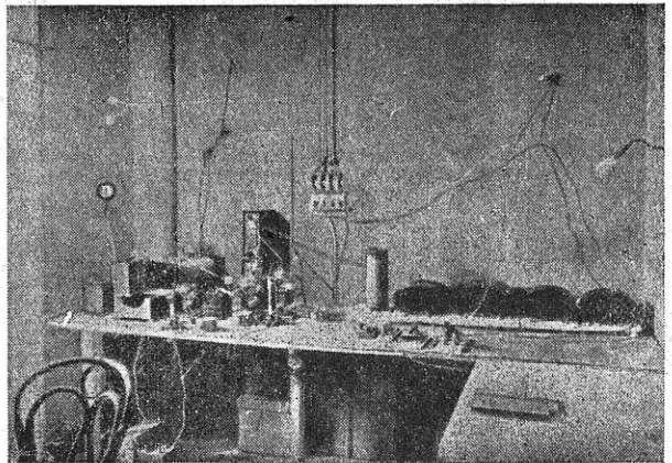
L. Deloy esimene lühilaine vastuvõtuseadeldis
