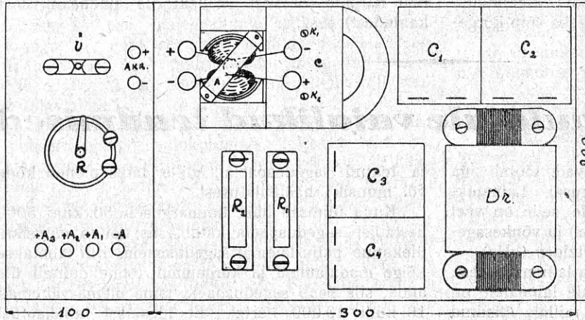
Montaasiskem.
