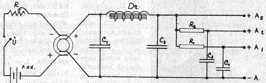
Üldskeem.
